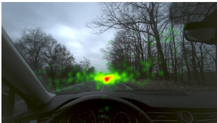
Obrázek 21 Heatmapa řidič 2
