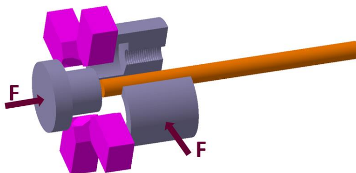
Obr. 22 Kování na vodorovných kovacích strojích. Přejato z [7]
