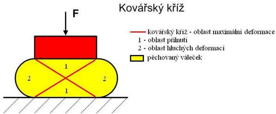
Obr. 10 Kovářský kříž. Přejato z [5, 6]
