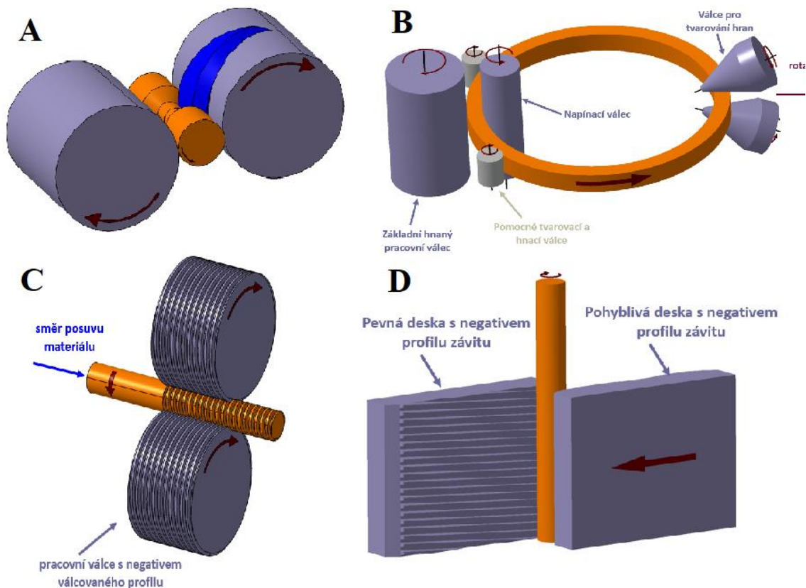
Obr. 33 A-Přičné klínové válcování, B-Válcování prstence, C-Podélné válcování závitů, D-Válcování závitu pomocí desek. Upraveno dle [9]
