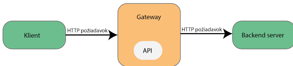
Obr. 3.6: Schéma API.
