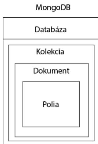
Obr. 3.10: Štruktúra MongoDB.
