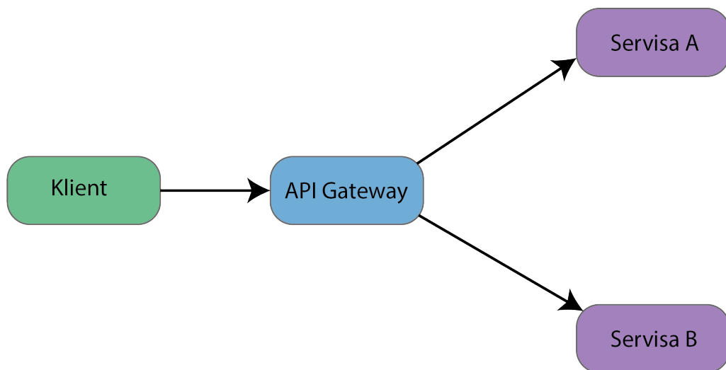
Obr. 3.5: Schéma mikroservisov.
