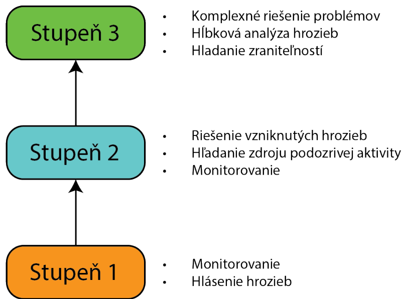
Obr. 2.1: Hierarchia SOC.
