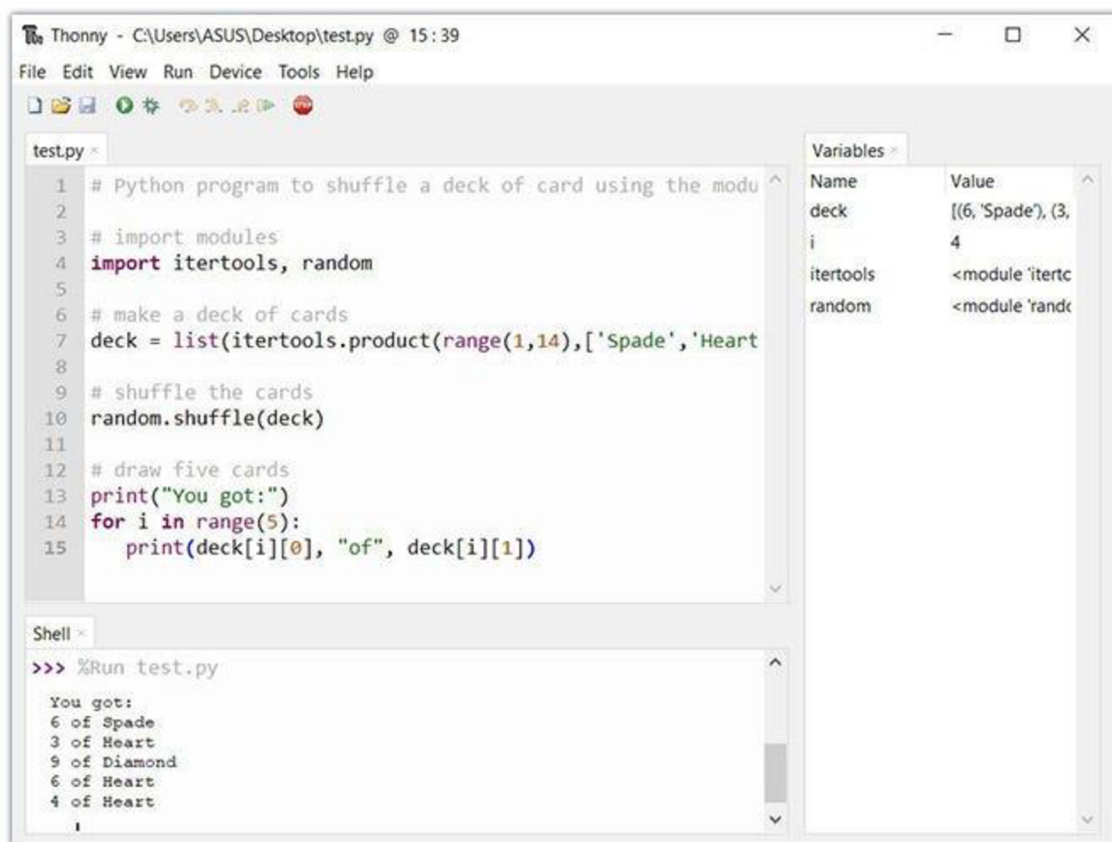
Obrázek 2 Thonny IDE [7]
