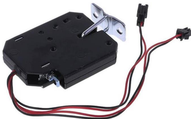
Obrázek 18 Elektromagnetický zámek [29]
