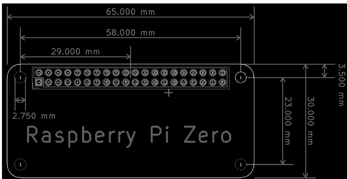
Obrázek 11 Rozměry Raspberry Pi Zero2 W [22]
