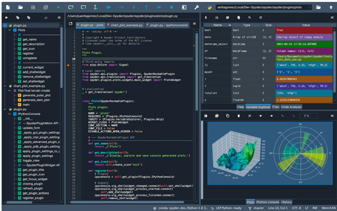
Obrázek 3 Spyder3 IDE [8]
