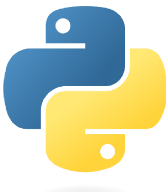
Obrázek 5 Python logo [15]
