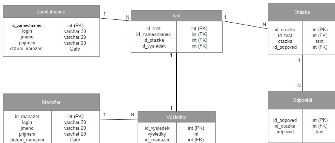
Obrázek 3: Relační model
