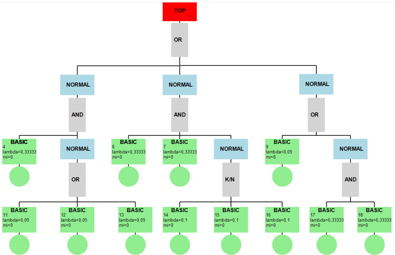
Příloha 1: Ukázka testovacího příkladu
