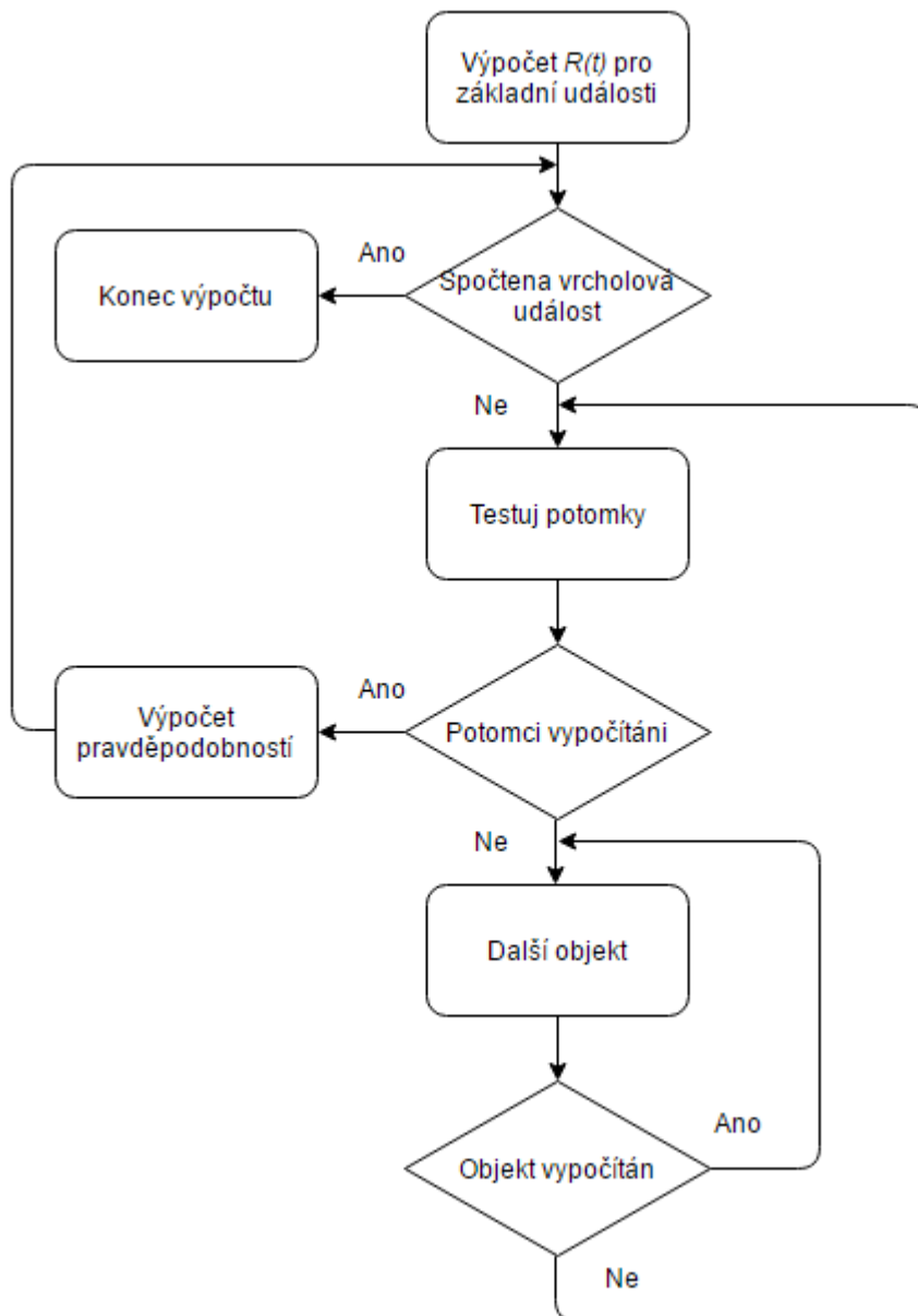
Obrázek 12: Algoritmus pro výpočet hodnot pravděpodobnosti bezporuchového provozu (prohledávání stromu do hloubky)
