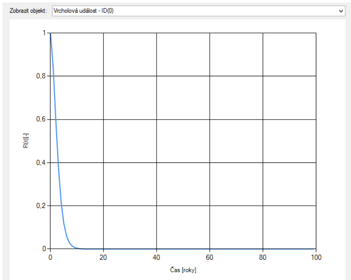
Příloha 3: Výsledný graf vrcholové události testovacího příkladu
