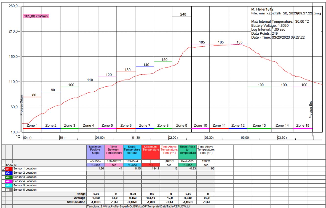
Obrázek 15: Teplotní profily
