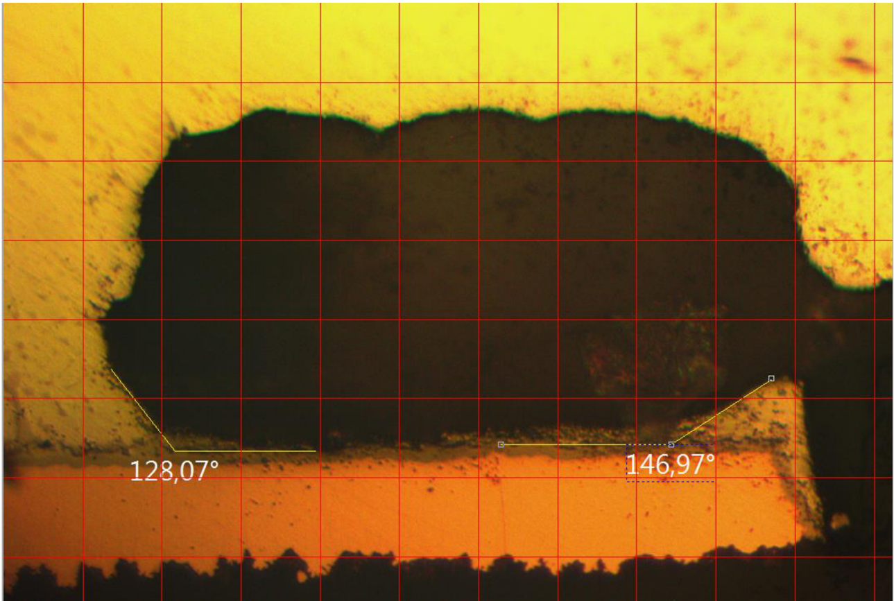
Obrázek 36: Měření úhlů u defektu (voidu)
