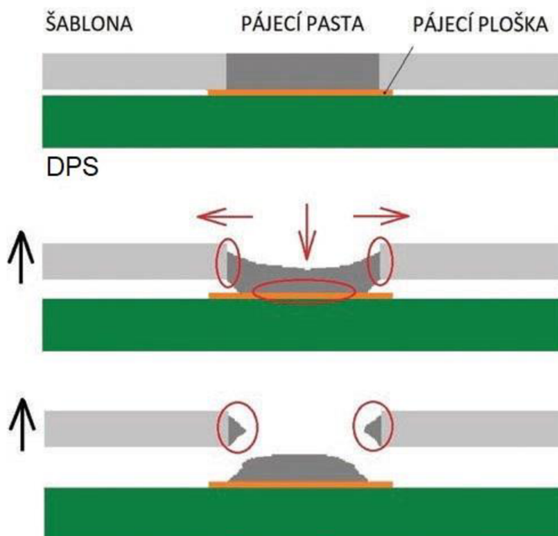
Obrázek 2: Šablonový tisk
