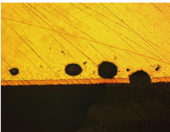
Obrázek 34: Vzorek 3_2 2.V po celém cyklu stárnutí detail mezery
