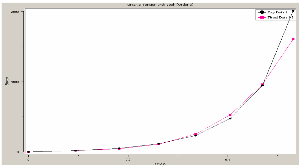
Obr. 6.4 – aproximace křivky \sigma – \epsilon odpovídající adverticii pomocí modelu Yeoh 3. řádu [kPa]
