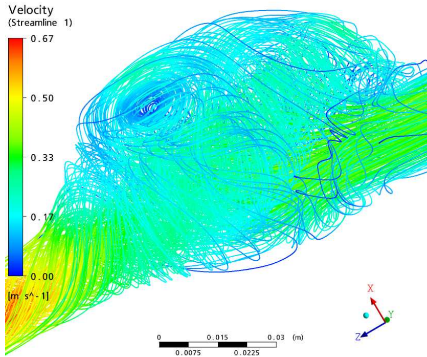
Obr. 7.10 – rychlostní pole ve formě proudnic [m/s]
