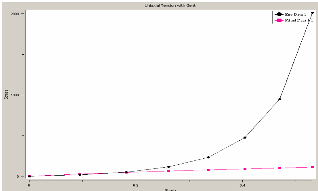
Obr. 6.3 – aproximace křivky \sigma – \epsilon odpovídající adverticii pomocí modelu Gent [kPa]
