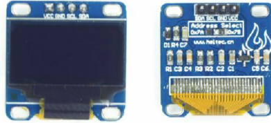
Obr. 2.3: Informační displej IIC I2C OLED.
