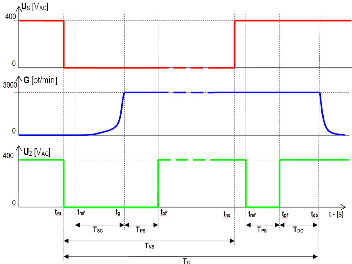
Obrázek 48. Ovládání motorgenerátoru - základní režimy a časový průběh při výpadku sítě.
