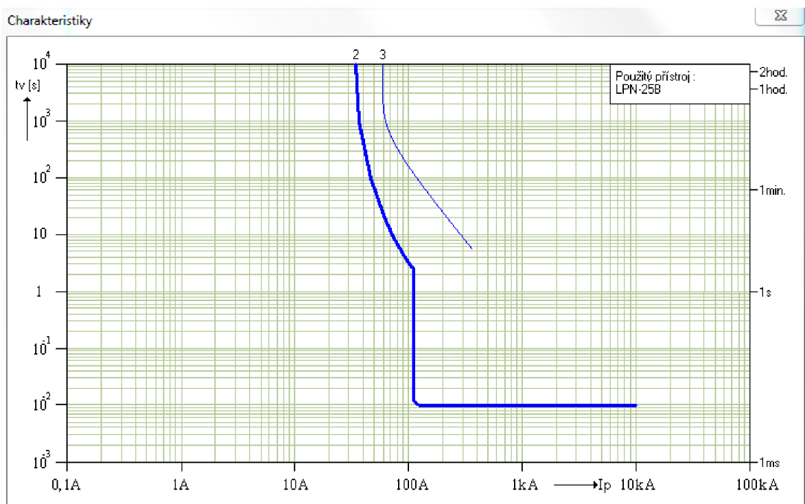
Obrázek 44. Vypínací charakteristika - selektivita jištění.
