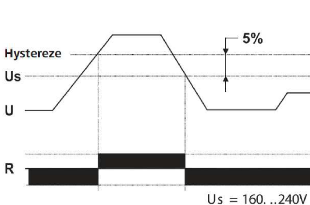
Obrázek 31. Časový průběh 3f relé.
