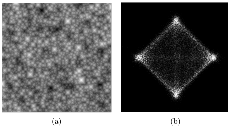
Obr. 3.6: a) Počítačovo simulovaný povrch solárneho článku b) Rozptylový obraz tohto povrchu vypočítaný v rámci skalárnej Kirchoffovej teórie rozptylu.
