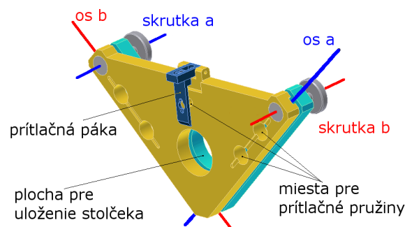
Obr. 5.2: Perspektívny pohľad na stolček
