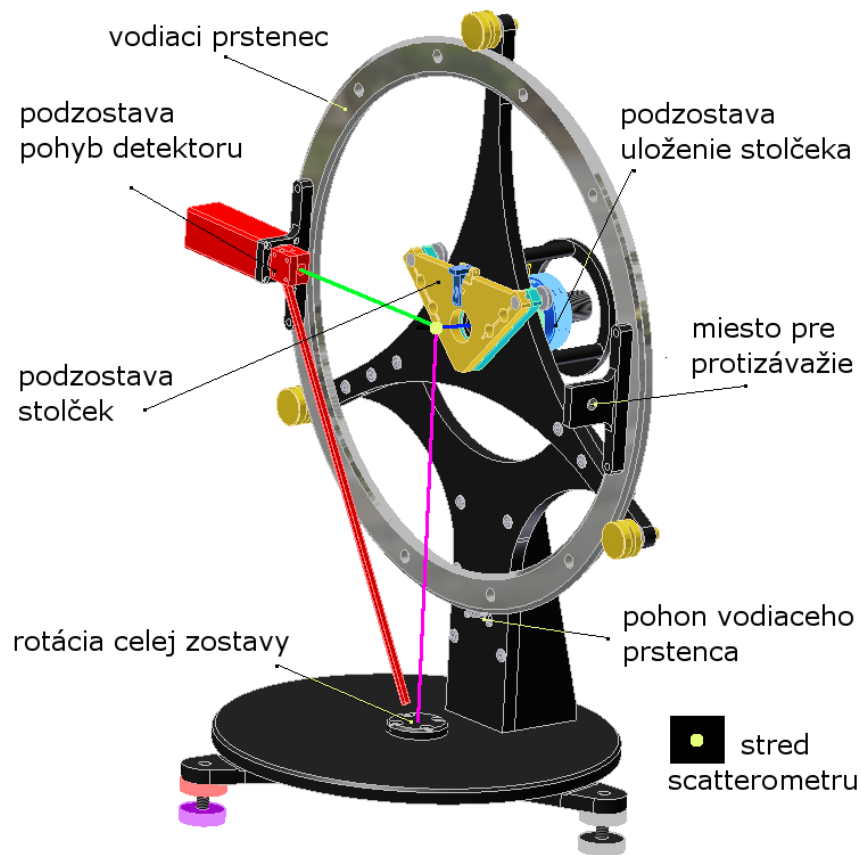
Obr. 5.1: Schéma Scatterometru
