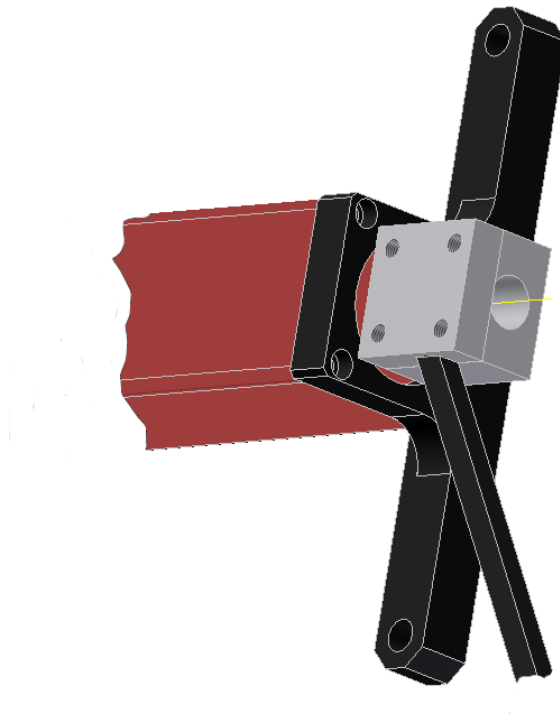
Obr. 5.5: Uchytenie motoru a ramienka s diódou
