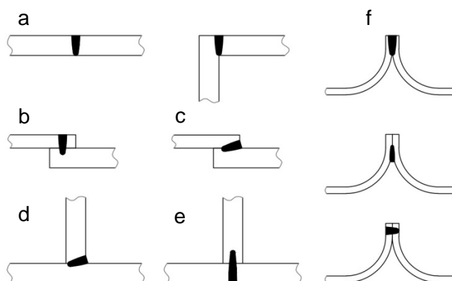
Obr. 2. 10: Možnosti provedení svarů a. Plochý I spoj, b. Svar přeplátovaného spoje, c. Koutový svar přeplátovaného spoje, d. Koutový svar T spoje, e. Provedení T spoje, f. Lemové svary na přírubě [4]
