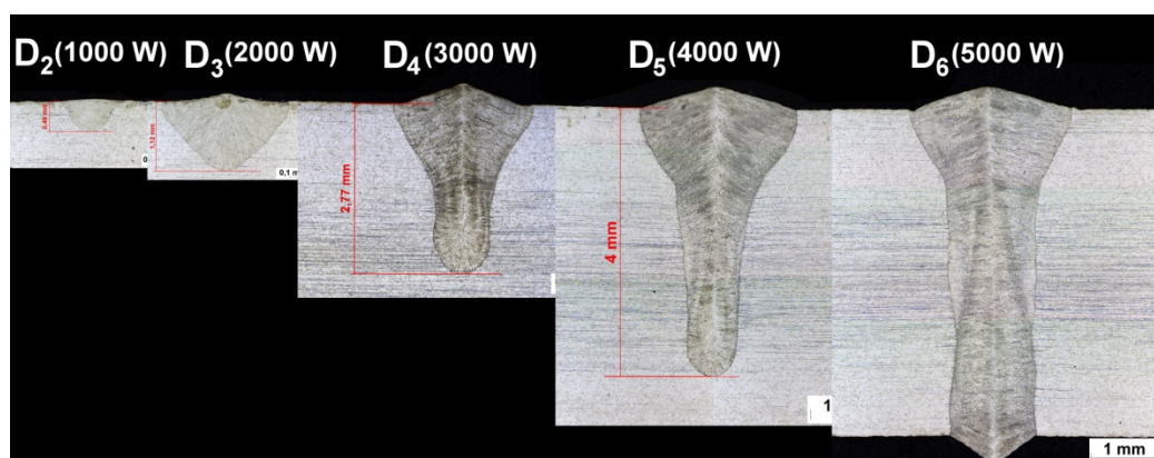
Obr. 5.19: Vzorky vytvořené rychlostí 2000 [mm/min] při zvyšujících se výkonech
