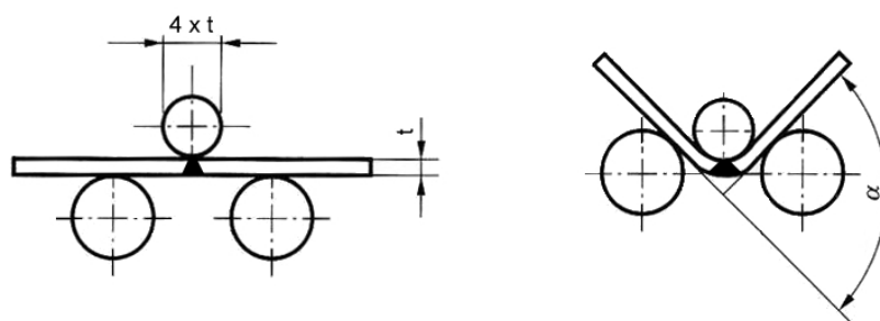
Obr. 3.8: Zkouška lámavosti [22]
