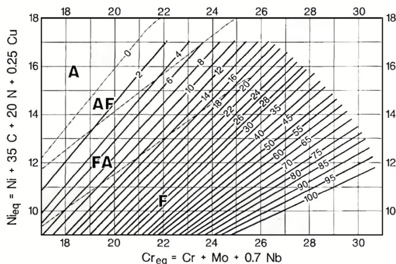
Obr. 4. 4: WRC-1992 diagram [28]
