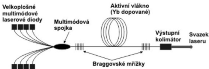
Obr. 2. 6: Schéma vláknového laseru [3]
