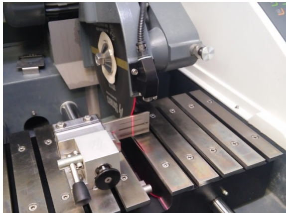
Obr. 5.13: Vyřezávání proužků k metalografii
