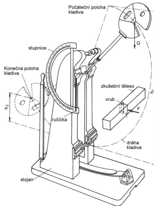
Obr. 3.9: Charpyho kladivo [23]
