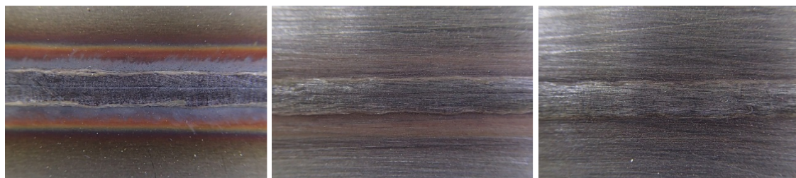
Obr. 5. 28: Snímky líce svarového spoje
