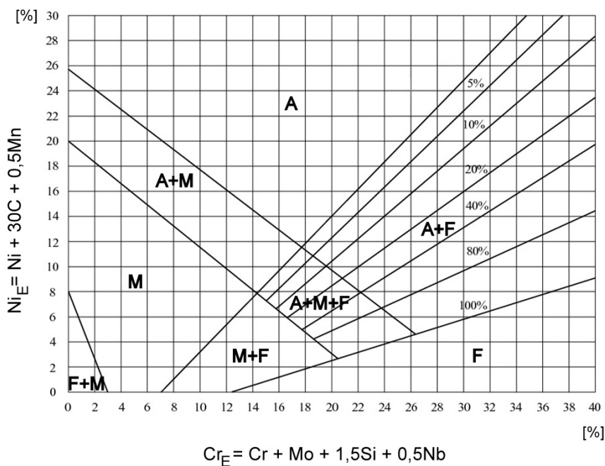
Obr. 4. 2: Schaefflerův diagram [27]
