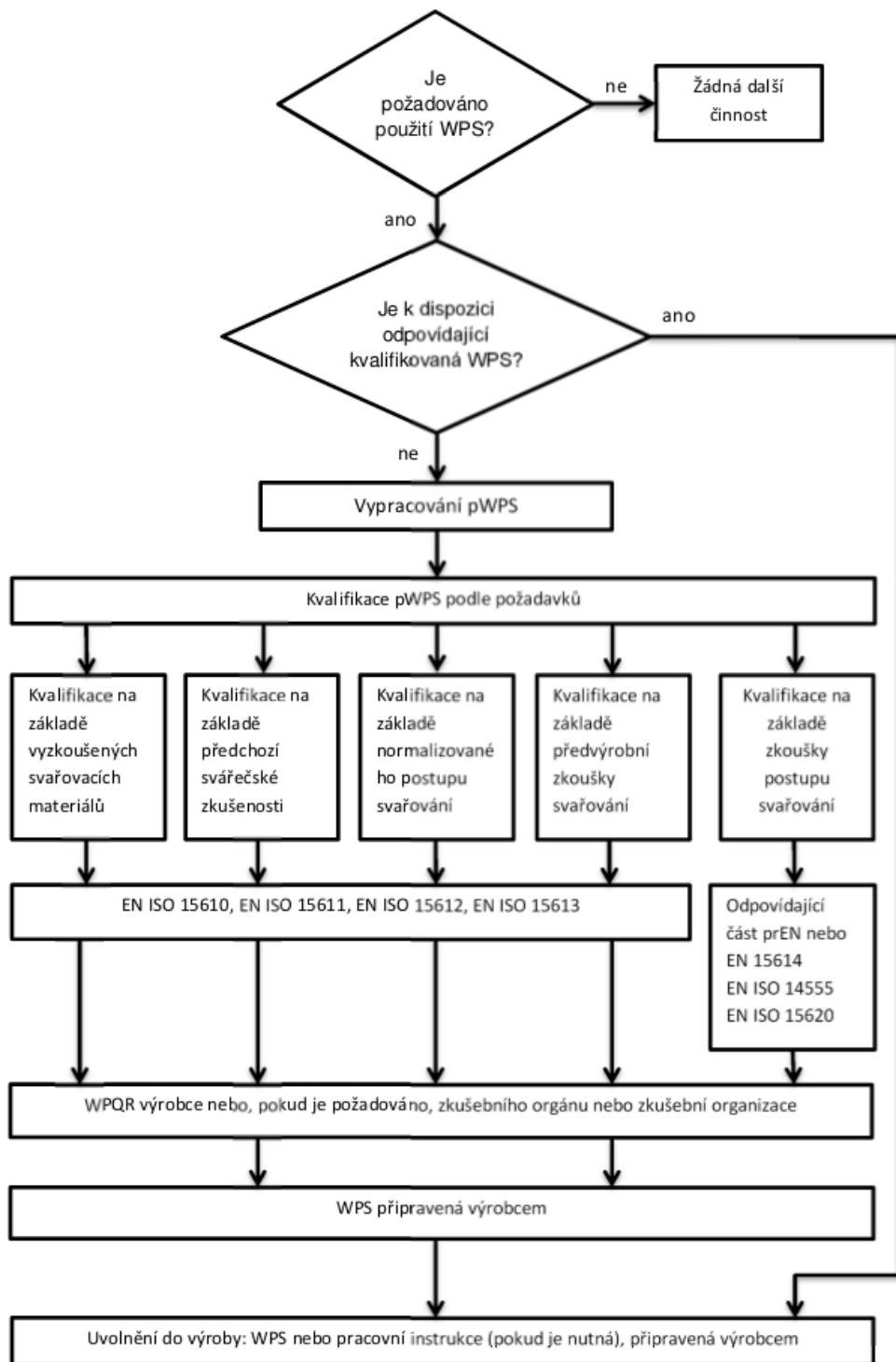
Obr. 3. 1: Postupový diagram pro vypracování a kvalifikaci WPS [11]
