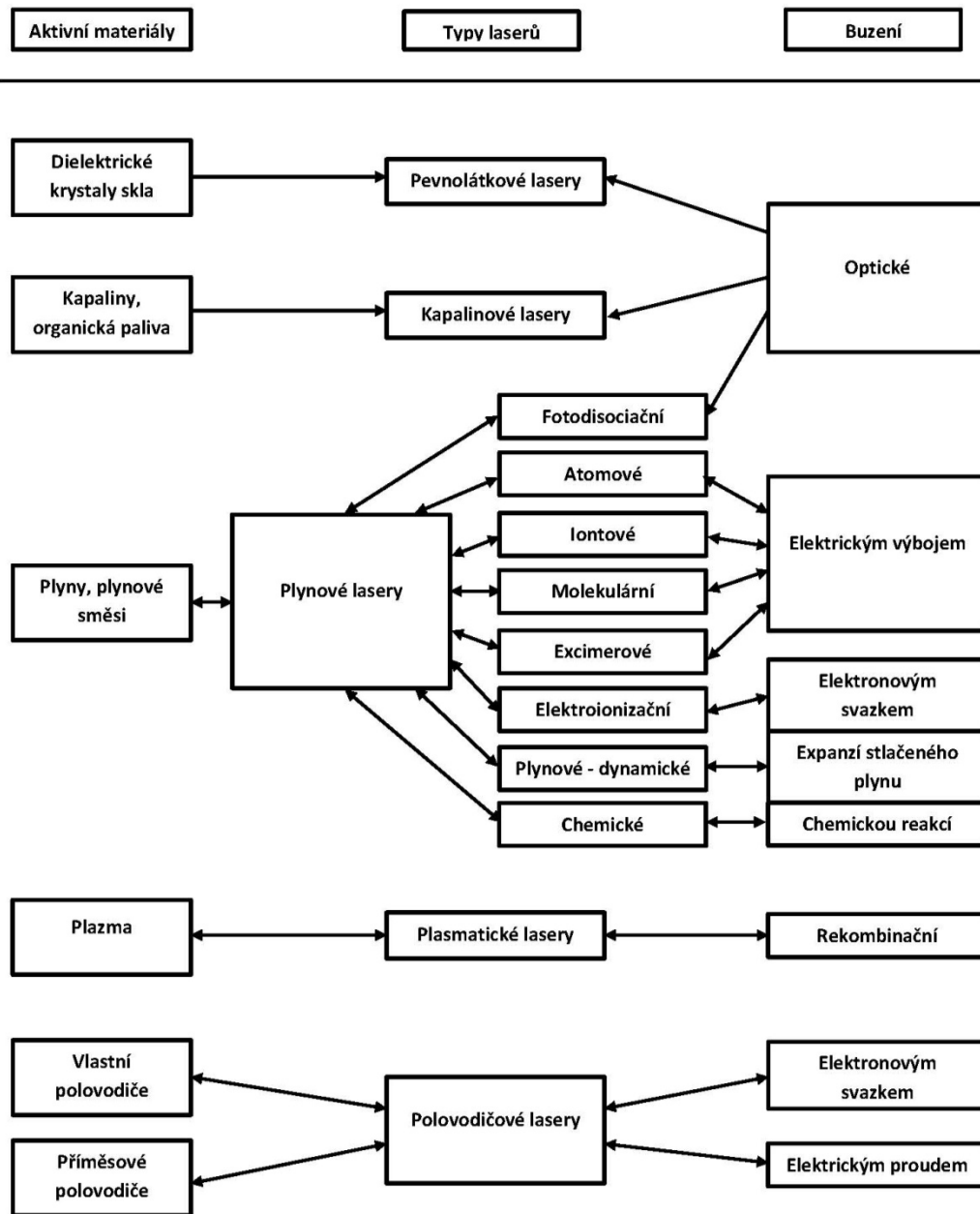
Obr. 2. 3: Rozdělení laserů [5]
