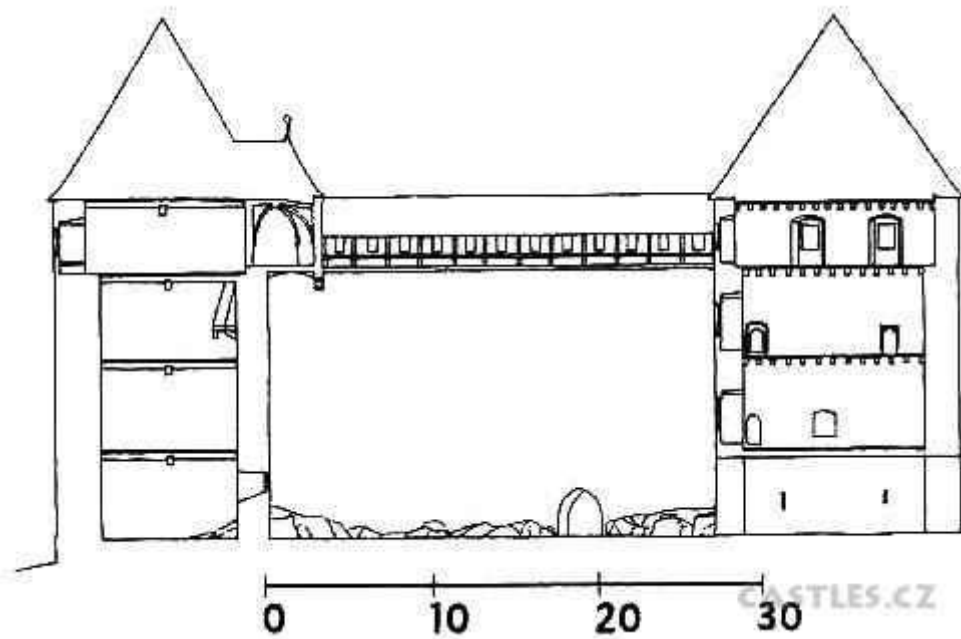
11. Řez obytným jádrem hradu – jižní pohled (podle D. Menclové)
