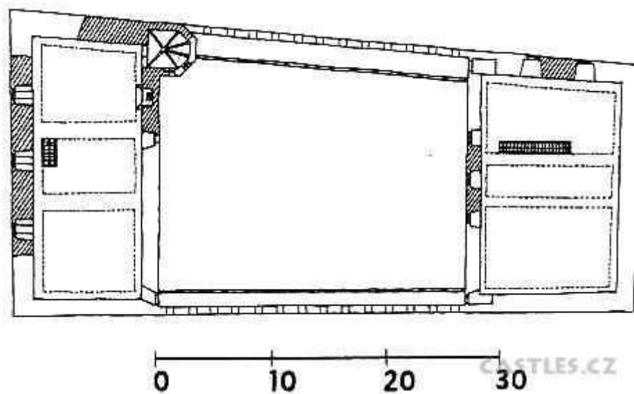
15. Půdorys 3. patra obytného jádra (podle D. Menclové)
