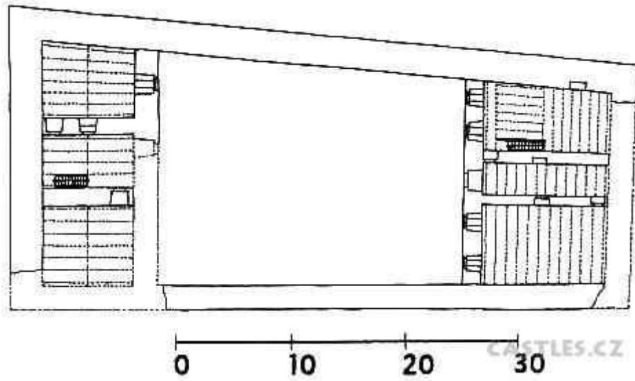
13. Půdorys 1. patra obytného jádra (podle D. Menclové)
