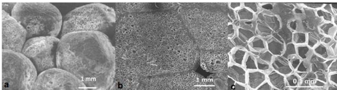
Obrázek 10: Struktura EPS pod elektronickým mikroskopem – a) perle, b) rozříznuté perle a uzavřené buňky, c) uzavřené buňky [43]
