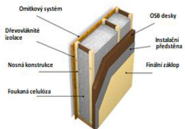
Obrázek 6: Skladba lehké neovětrávané obvodové stěny [37]
