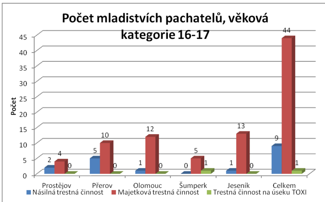
Graf č. 3 Souhrnný histogram relativních četností
