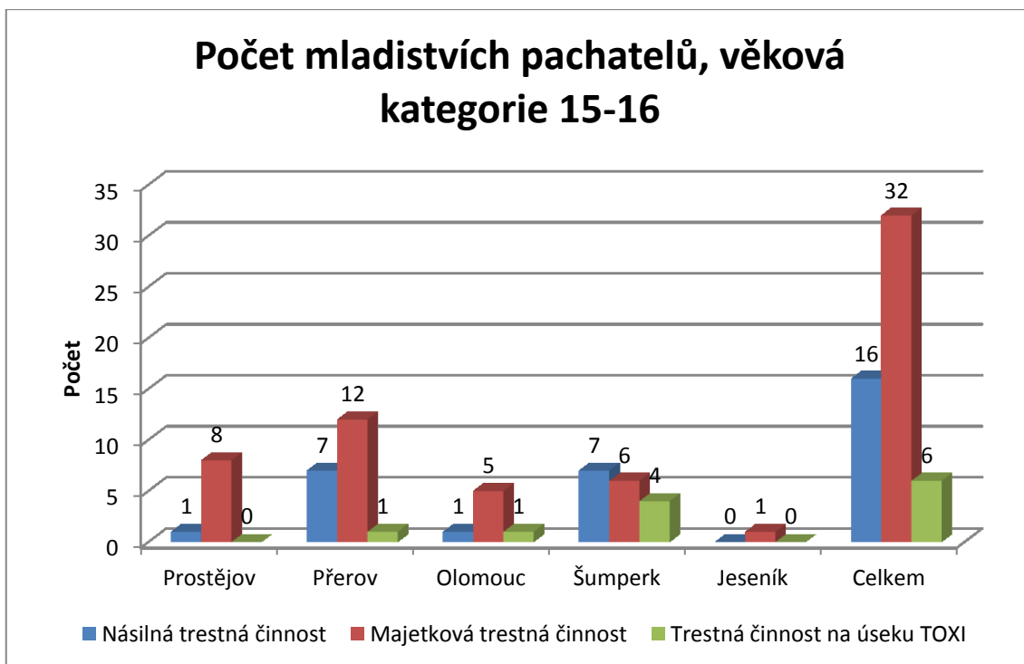
Graf č. 2 Souhrnný histogram relativních četností
