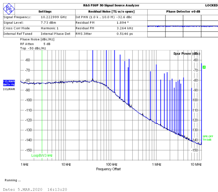
Obrázek 28 Fázový šum signálu 12 GHz při proudu nábojové pumpy I_{CP} = 5,549 mA, low-noise mód, interní reference
