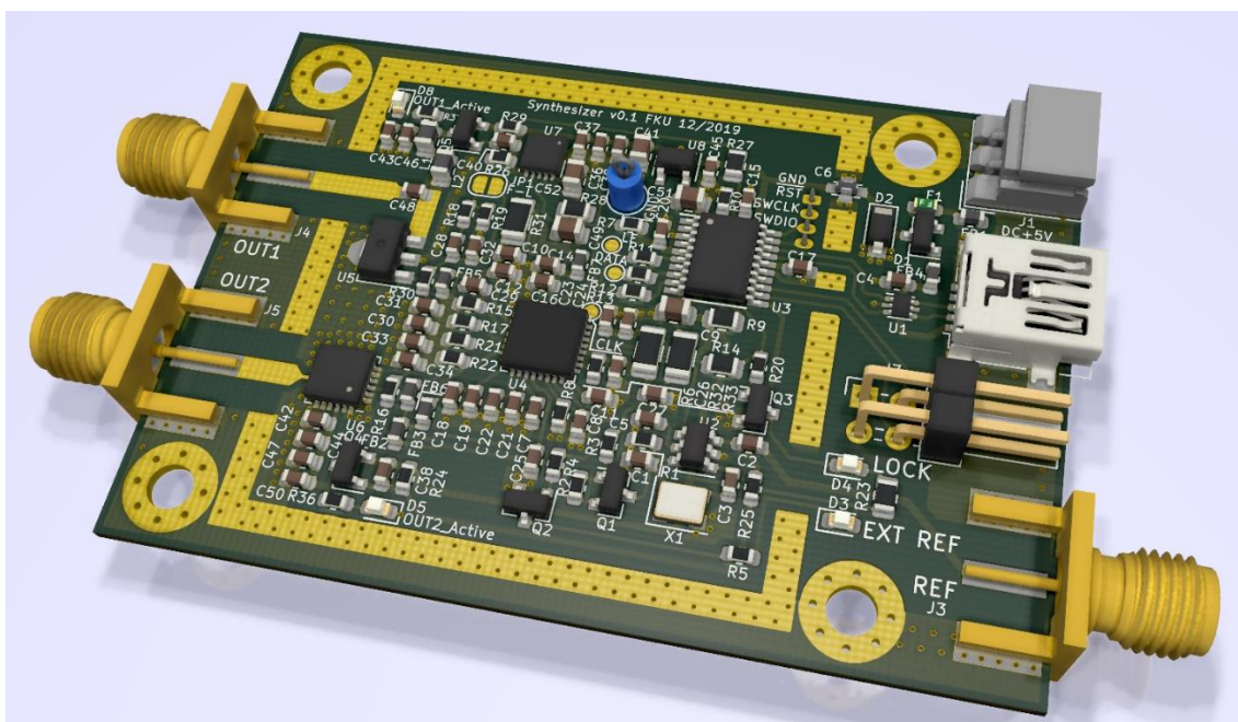
Obrázek 16 3D vizualizace návrhu realizace frekvenčního syntezátoru
