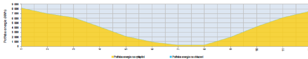
GRAF: Potřeba energie na vytápění a chlazení podle ČSN EN ISO 13786
