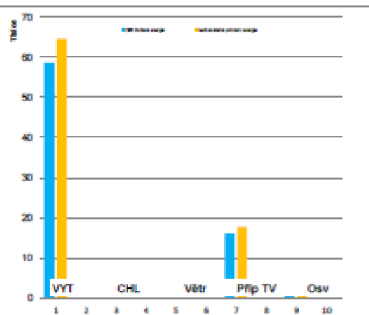
GRAF: Dílčí dodaná energie, neobnovitelná primární energie pro hodnotenou budovu
