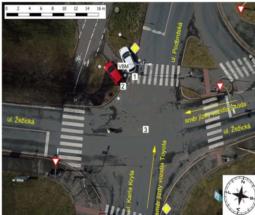
Obr. č. 4 – Plánek dopravní nehody č. 4 - autor nrap. Radek Hampejs
