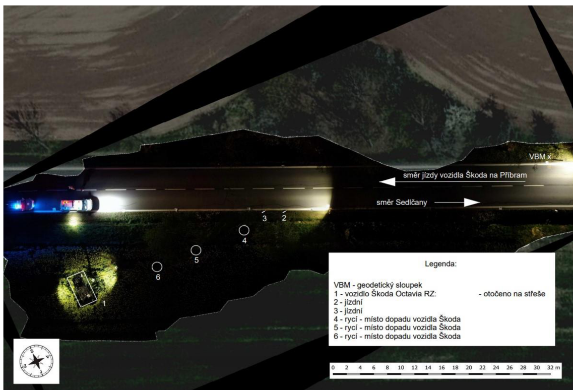
Obr. č. 1 – Plánek dopravní nehody č. 1 - autor nrap. Radek Hampejs
