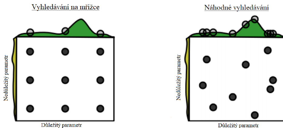
Obrázek 14 – Porovnání náhodného hledání s hledáním na mřížce [29]
