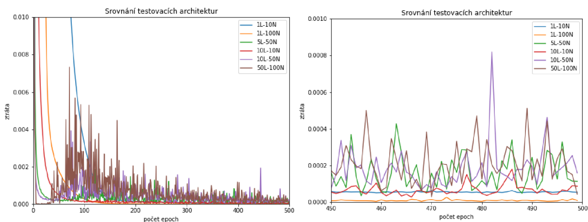
(a) Výkony testovacích sítí
