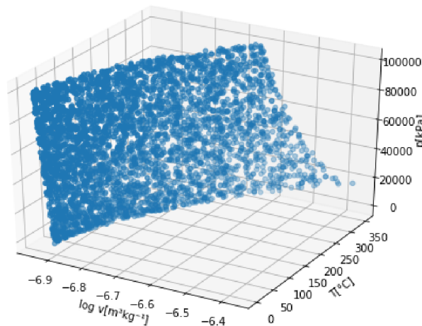
Obrázek 17 – Vygenerovaná data
