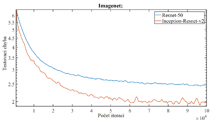
Obrázek 5 – Ukázka underfittingu [8]
