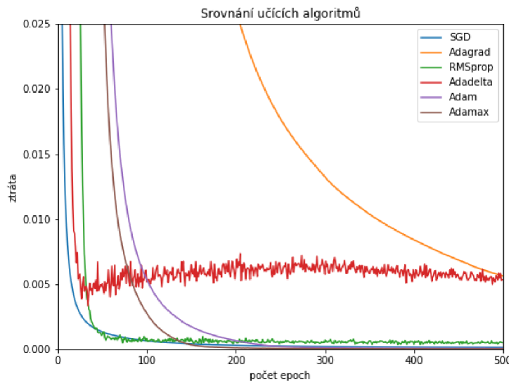
Obrázek 18 – Srovnání algoritmů
