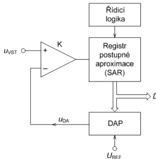
Obr. 4.1: Schema kompenzačního A/D převodníku s postupnou aproximací. [15]
