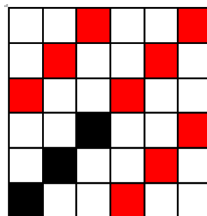
Obrázek 7. Keprová vazba
