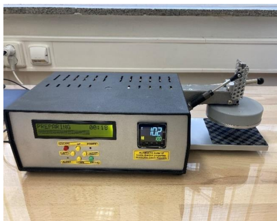
Obrázek 2. Alambeta
