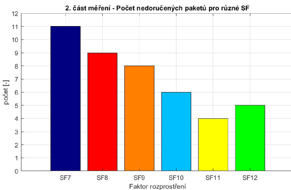
Obr. A.11: Graf množství nedoručených paketů z celkového počtu 16 pro každý uvedený SF - 2. část měření
