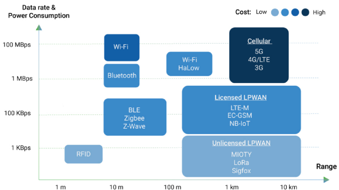
Obr. 1.4: Srovnání IoT bezdrátových technologií v závislosti na dosahu komunikace, rychlosti přenosu dat a spotřebě energie [27]
