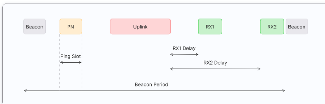
Obr. 2.9: Průběh komunikace zařízení třídy B [1]
