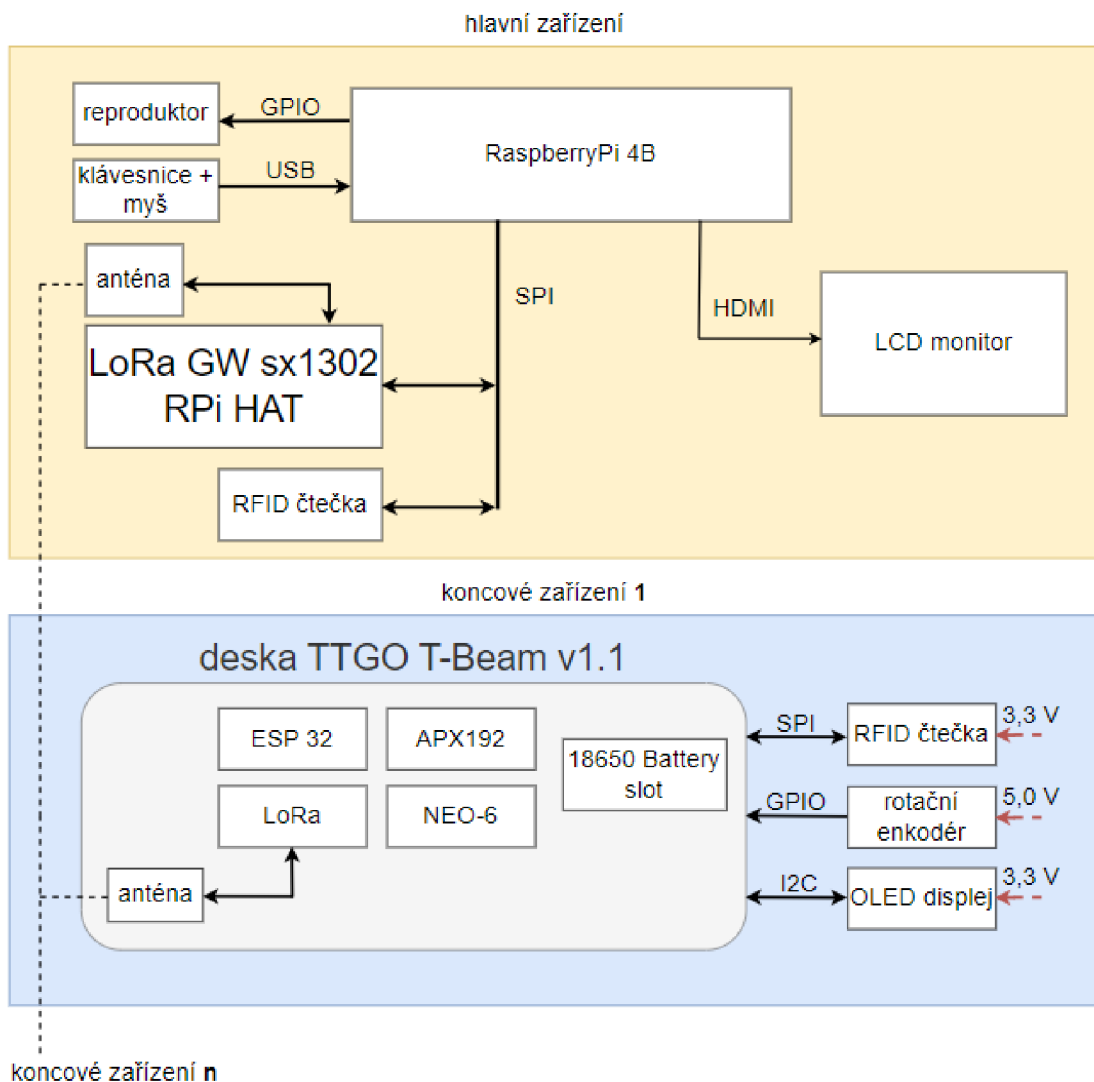
Obr. 3.2: Blokové schéma zapojení zařízení v síti
