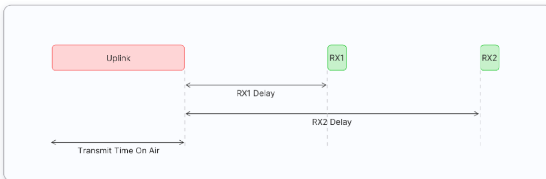
Obr. 2.8: Průběh komunikace zařízení třídy A [1]
