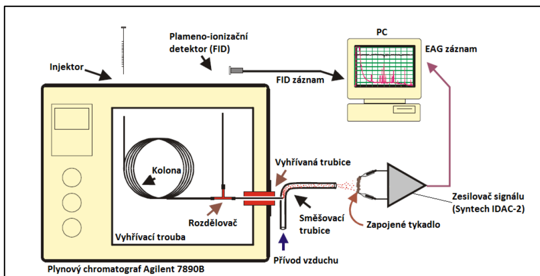
Obrázek 3: Schéma zapojení plynové chromatografie s elektroantenografickou detekcí GC -EAD. Zdroj: Syntech (2004)
