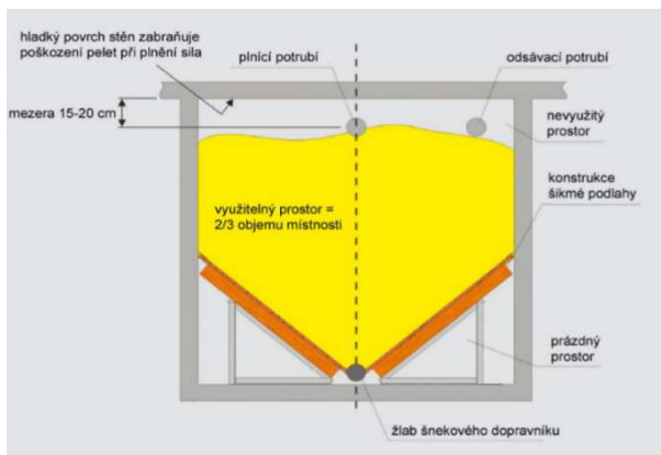
Obrázek 14 Konstrukce skladu [11]
