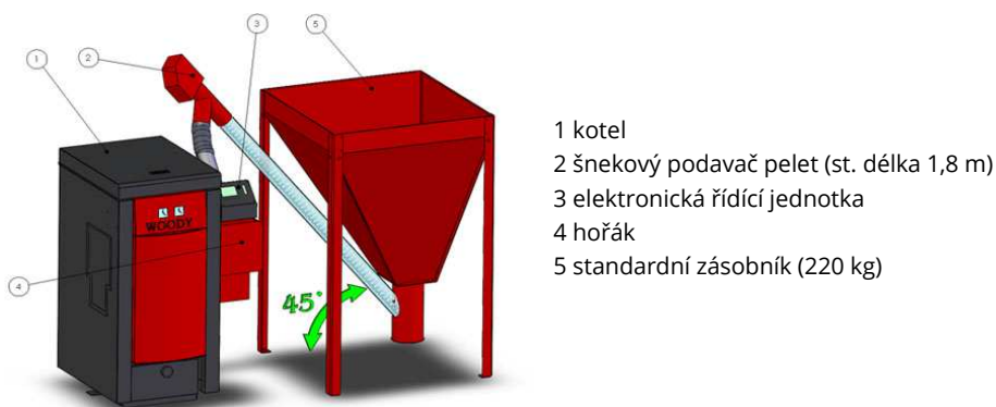
Obrázek 9 Peletový kotel se standardním zásobníkem pro 220 kg pelet a se standardní délkou šnekového podavač 1,8 m [8]
