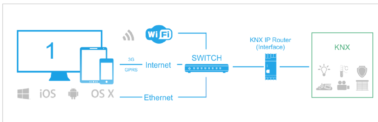
Obr. 32) Schéma připojení při použití obyčejného KNX/IP routeru
