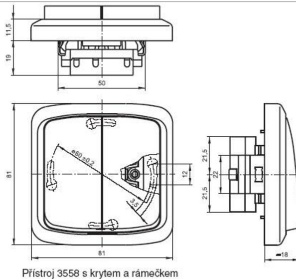
Přístroj 3558 s krytem a rámečkem
