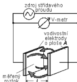
Obr. 9: Schéma měření vodivosti roztoků [24]
