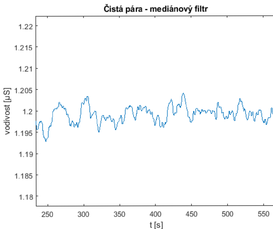
Obr. 34: Detail signálu snímané vodivosti
