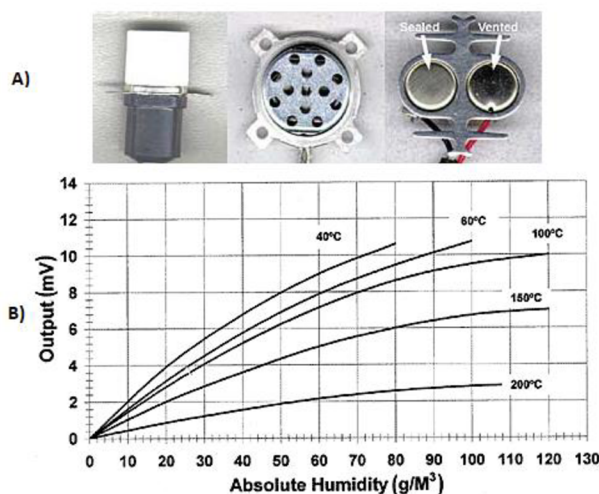
Obr. 8: A: Vlhkoměr s vyhřívajícími termistory, B: Závislost absolutní vlhkosti na teplotě a napětí [23]
