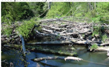
Kenická akumulace -2007 (Máčka, Krejčí, 2011)
