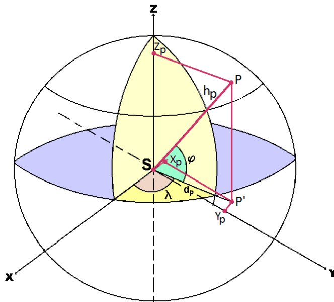
Obr. 6.1 Parametry elipsoidu pro definovaný bod \mathbf{P} .
