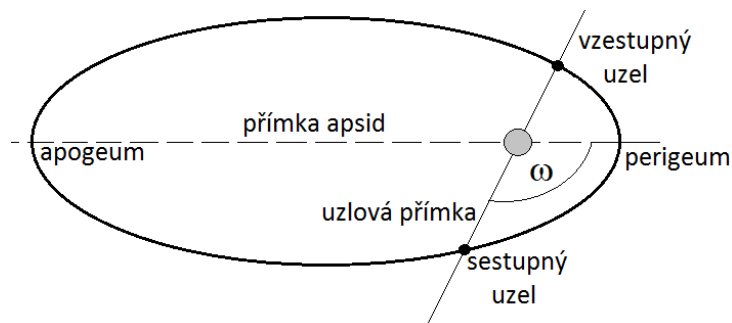
Obr. 7.2: Určení argumentu perigea.
