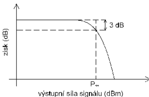
Obr. 3.6: Graf závislosti síly výstupního signálu na zisku polovodičového OZ.
