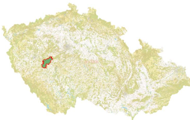
Obr. 4 Vyznačené území CHKO Brdy
