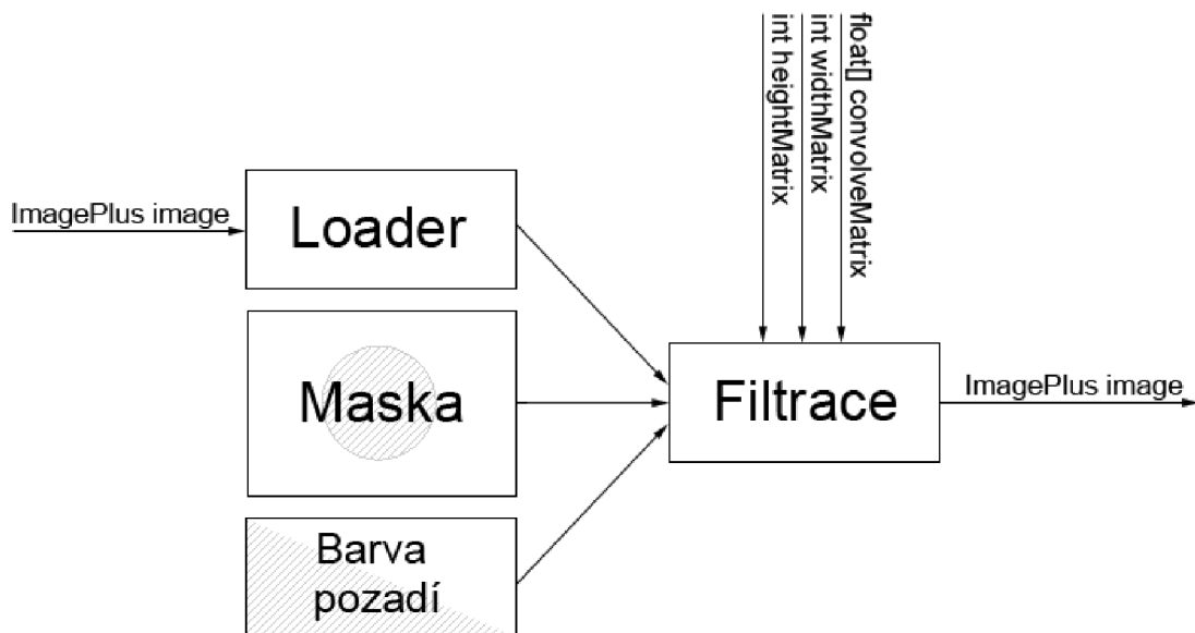
Obrázek 5.15: Komponenty pro začlenění do evolučního systému
