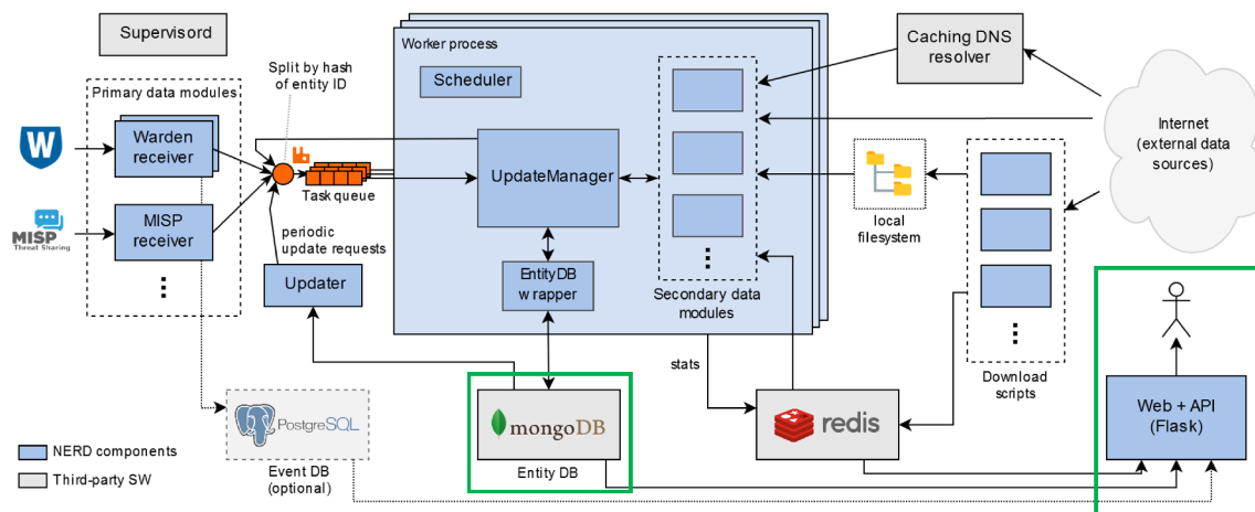
Obr. 2.1: Architektúra systému NERD prevzatá z [2]
