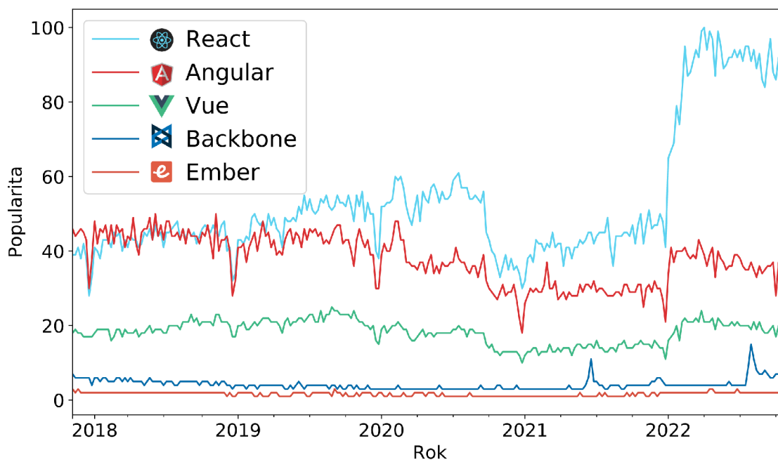
Obr. 2.2: Popularita frameworkov JavaScript za posledných 5 rokov získaná z dát Google Trends [11] dňa 09.11.2022
