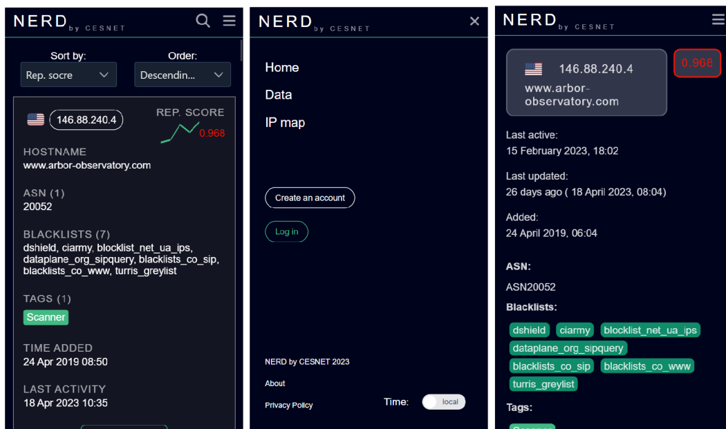
Obr. 3.24: Ukážka zobrazenia na mobilných zariadeniach: hlavná stránka (vľavo), mobilné menu (v strede) a detail IP adresy (vpravo)
