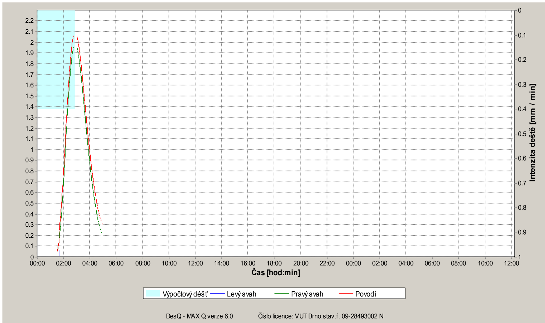
Graf 5-1 Průběh povodňové vlny v zájmovém povodí – program DesQ - MaxQ.
