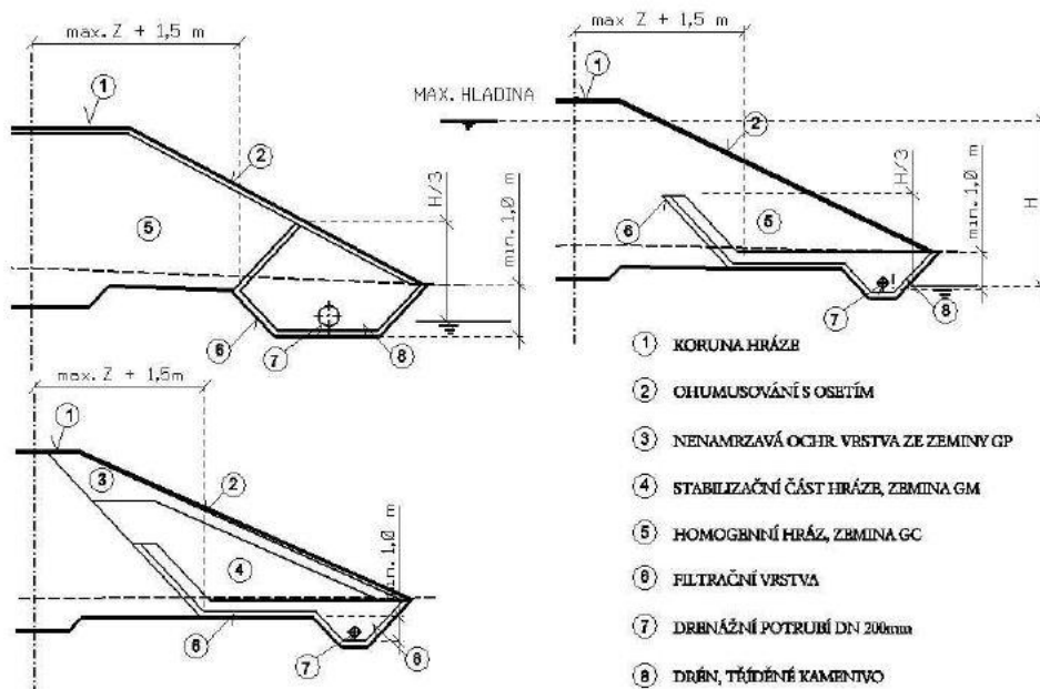
Obr. 6-3 Ukázka patních drénů [5].
