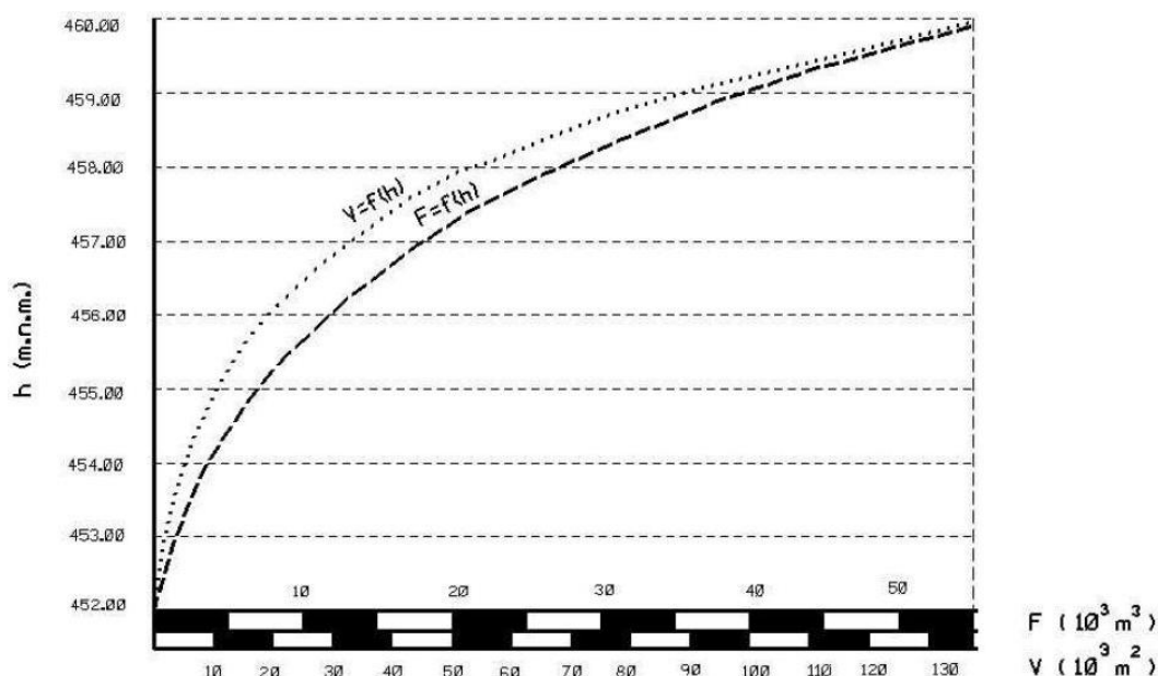
Obr. 5-3 Batygrafické čáry nádrže [5].
