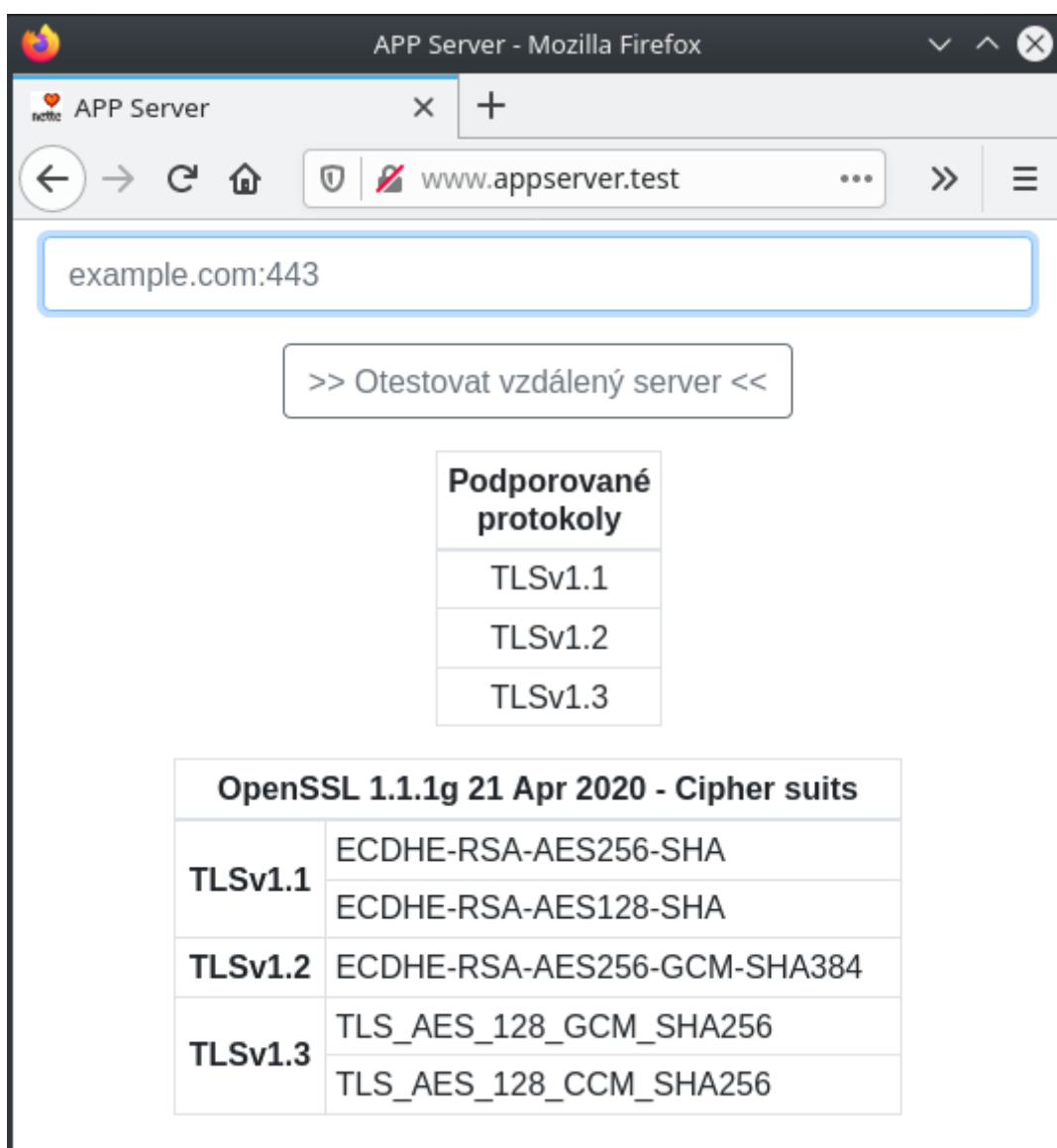
Obr. 2.4: Grafická podoba webu po výstupu prvního skriptu.
