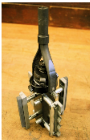
Obrázek 1.1 Honovací hlava
