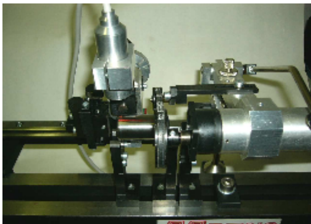
Obrázek 3.29 Nastavení měřicího přístroje při měření vad na válcové ploše
