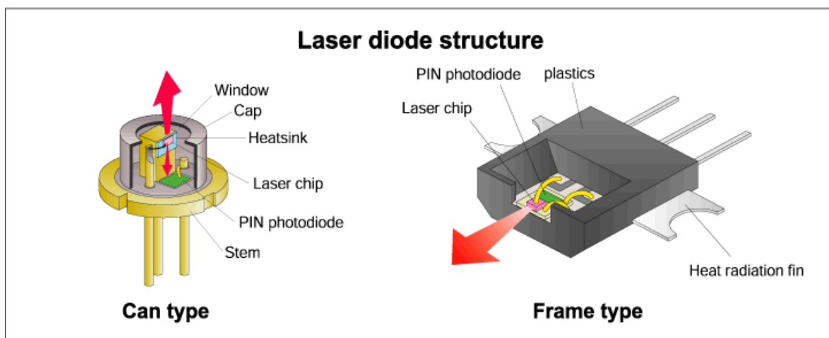
Obrázek 3.20 Základní typy polovodičových laserů
