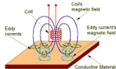
Obrázek 2.15 Vytváření vířivých proudů v materiálu
