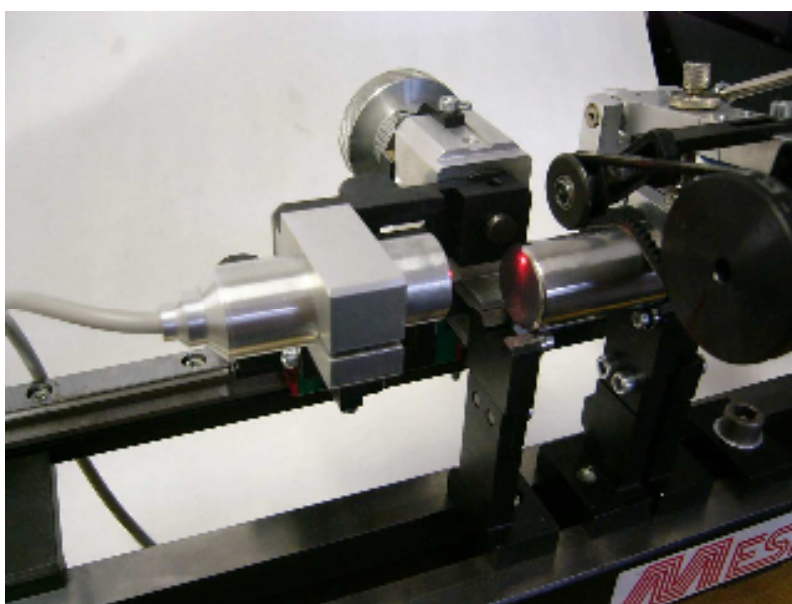
Obrázek 3.40 Nastavení měřícího přístroje při měření vad čelních ploch
