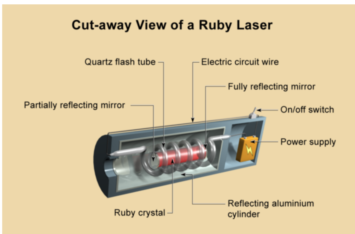
Obrázek 3.12 Schéma rubínového laseru
