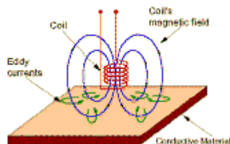
Obrázek 2.14 Vytváření magnetického pole cívkou
