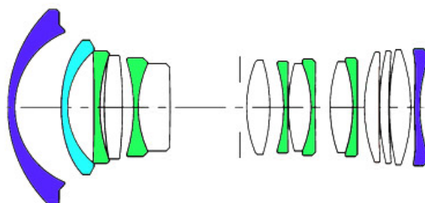
Obrázek 3.9 Uspořádání čoček v objektivu
