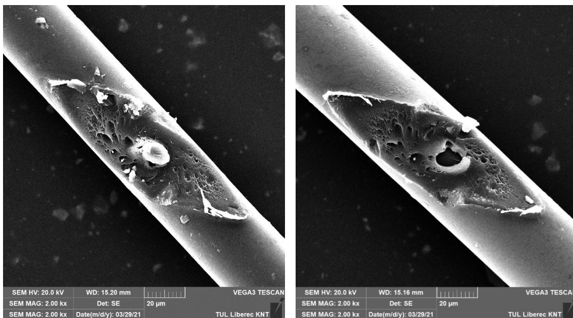
Obr. č. 20 - Vzniklá struktura po oddělení dvou bikomponentních vláken jejichž úhel pojení byl 29^\circ
