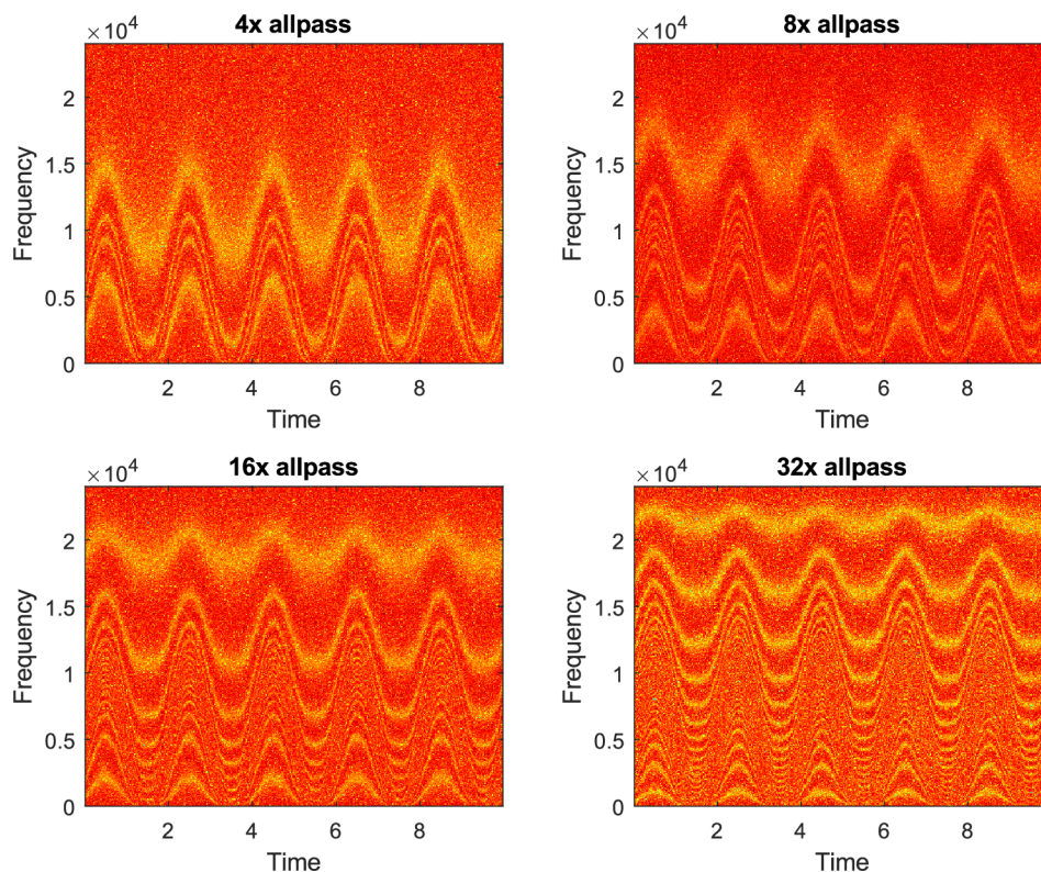
Obrázek 4.4: Phaser, odezva bílého šumu
