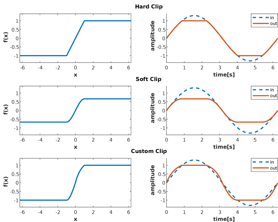
Obrázek 4.2: Ořezávací funkce
