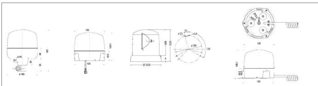
Obrázok 8 - Spôsoby upevnenia majákov [15]
