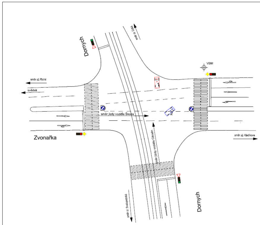
Obrázok 25 - Plánik miesta nehody Zdroj: PČR [45]
