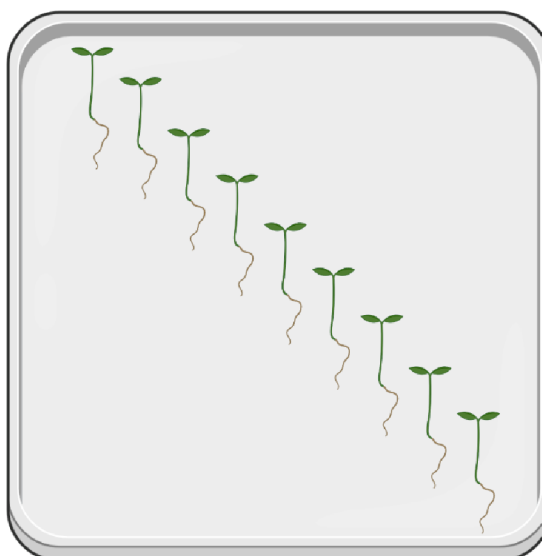
Obr. 11. Rozložení rostlin na agarovém MS médiu v hranatých Petriho miskách při fototropických experimentech.
