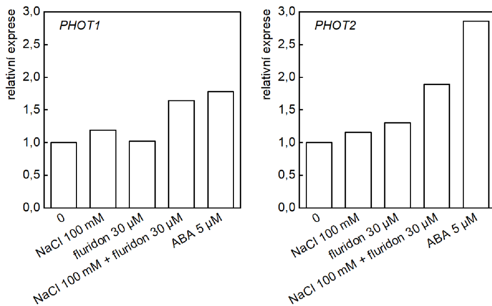
Obr. 31. Relativní exprese genů PHOT1 a PHOT2 v prýtech (hypokotylech a kotyledonech) osmidenních rostlin Arabidopsis , genotypu gl-1 po 24 hodinách kultivace na jednosměrném horizontálním modrém světle (BL) na agarovém MS médiu s obsahem NaCl o koncentraci 100 mmol l -1 , fluridonu o koncentraci 30 µmol l -1 , kombinace NaCl a fluridonu (stejně koncentrace jako při samostatné aplikaci) a exogenní ABA o koncentraci 5 µmol l -1 . Výsledky představují hodnoty relativní exprese (vztážené k housekeeping genu EF1α ) z jednoho samostatného experimentu vypočítané z průměrných Ct hodnot ze 3 technických replikátů z dané testované podmínky. Statistická analýza nebyla provedena z důvodu nízkého počtu experimentů.
