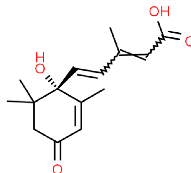
Obr. 6. Kyselina abscisová.
