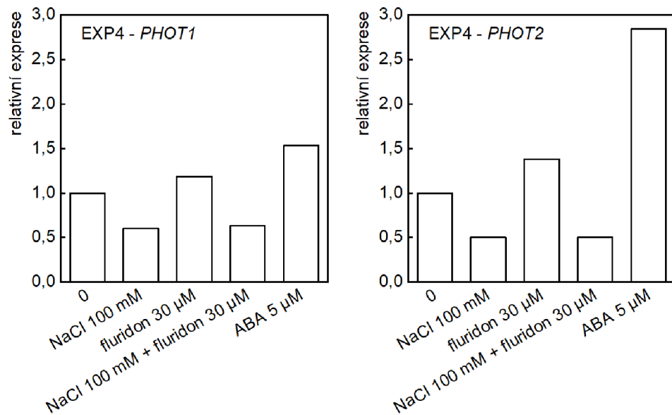
Obr. 33. Relativní exprese genů PHOT1 a PHOT2 v prýtech (hypokotylech a kotyledonech) osmidenních rostlin Arabidopsis , genotypu gl-1 po 24 hodinách kultivace na jednosměrném horizontálním modrém světle (BL) na agarovém MS médiu s obsahem NaCl o koncentraci 100 mmol l -1 , fluridonu o koncentraci 30 μmol l -1 , kombinace NaCl a fluridonu (stejně koncentrace jako při samostatné aplikaci) a exogenní ABA o koncentraci 5 μmol l -1 . Výsledky představují hodnoty relativní exprese (vztažené k housekeeping genu EF1α ) z reprezentativního experimentu (EXP4) vypočítané z průměru Ct hodnot ze 3 technických replikátů z dané testované podmínky. Statistická analýza nebyla provedena z důvodu nízkého počtu experimentů.
