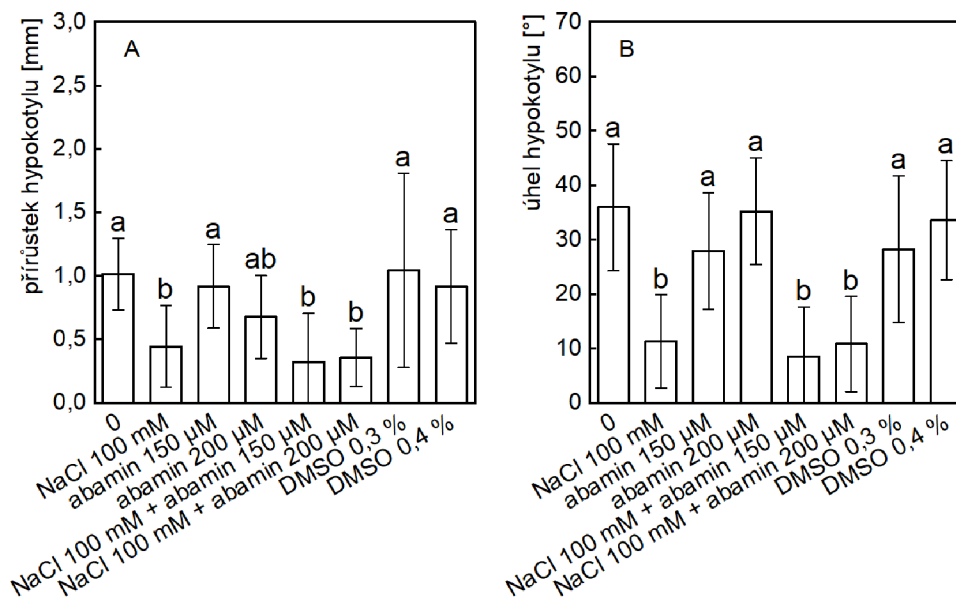
Obr. 26. Přírůstky [mm] (A) a fototropické úhly [°] (B) hypocotylů osmidenních rostlin Arabidopsis , genotypu gl-1 po 24 hodinách kultivace na jednosměrném horizontálním modrém světle (BL) na agarovém MS médiu s obsahem NaCl o koncentraci 100 mmol l -1 , abaminu o koncentraci 150 µmol l -1 s výslednou koncentrací DMSO 0,3 % (v/v) nebo o koncentraci 200 µmol l -1 s výslednou koncentrací DMSO 0,4 % (v/v) a kombinace NaCl a abaminu (stejně koncentrace jako při samostatné aplikaci) nebo čistého 0,3% (v/v) a 0,4% (v/v) DMSO. Výsledky představují průměrné hodnoty ± SD z naměřených hodnot jednotlivých rostlin samostatného experimentu. V experimentu bylo na jedné podmínce testováno 16 rostlin. Statisticky významné rozdíly mezi měřeními parametry jsou označeny pomocí abc systému – hodnoty, které nesdílí společné písmeno jsou statisticky významně odlišné (jednofaktorová ANOVA + Tukeyho test).
