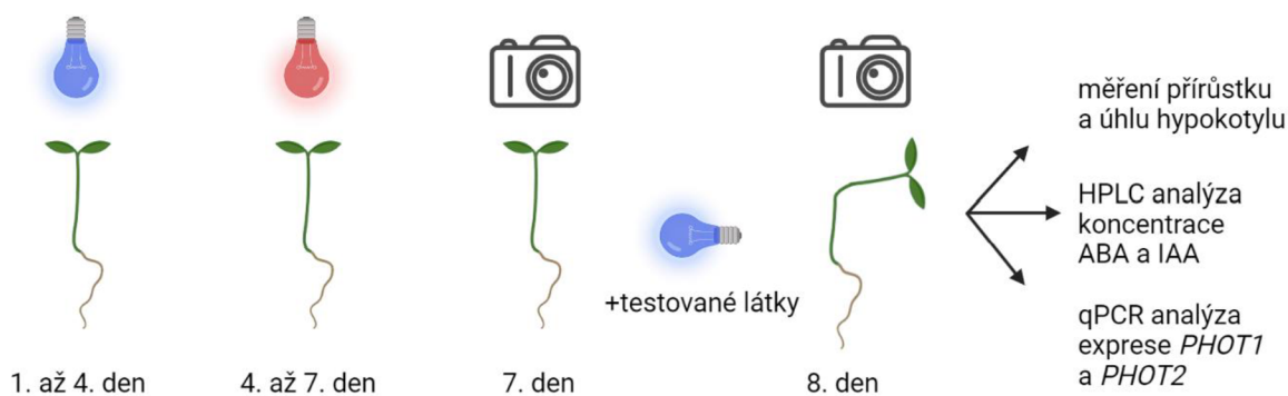
Obr. 12. Schéma průběhu fototropického experimentu s následnými analýzami.
