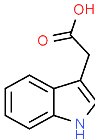
Obr. 5. Kyselina indol-3-octová (IAA).
