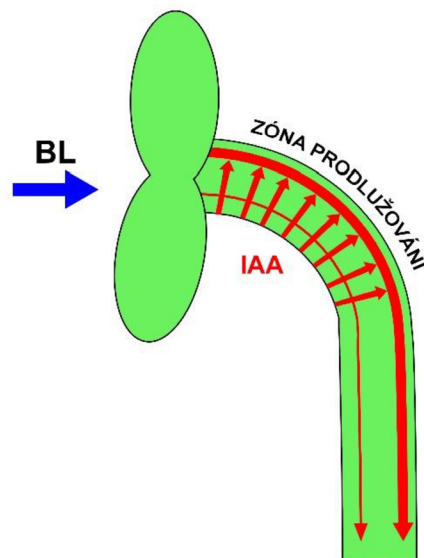
Obr. 4. Schéma fototropického ohybu hypokotylu. Modré světlo (BL) skrze signalizaci fototropinů způsobuje změny v proudění růstového hormonu auxinu (červené šipky), který následně způsobuje větší prodlužování buněk na neozářené straně. Podle Liscum et al., 2014).
