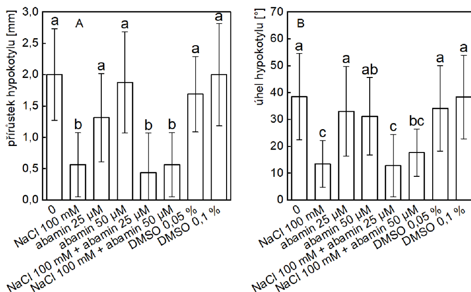
Obr. 25. Přírůstky [mm] (A) a fototropické úhly [°] (B) hypocotylů osmidenních rostlin Arabidopsis , genotypu gl-1 po 24 hodinách kultivace na jednosměrném horizontálním modrém světle (BL) na agarovém MS médiu s obsahem NaCl o koncentraci 100 mmol l -1 , abaminu o koncentraci 25 µmol l -1 s výslednou koncentrací DMSO 0,05 % (v/v) nebo o koncentraci 50 µmol l -1 s výslednou koncentrací DMSO 0,1 % (v/v) a kombinace NaCl a abaminu (stejné koncentrace jako při samostatné aplikaci) nebo čistého 0,05% (v/v) a 0,1% (v/v) DMSO. Výsledky představují průměrné hodnoty ± SD z naměřených hodnot jednotlivých rostlin samostatného experimentu. V experimentu bylo na jedné podmínce testováno 16 rostlin. Statisticky významné rozdíly mezi měřeními parametry jsou označeny pomocí abc systému – hodnoty, které nesdílí společné písmeno jsou statisticky významně odlišné (jednofaktorová ANOVA + Tukeyho test).
