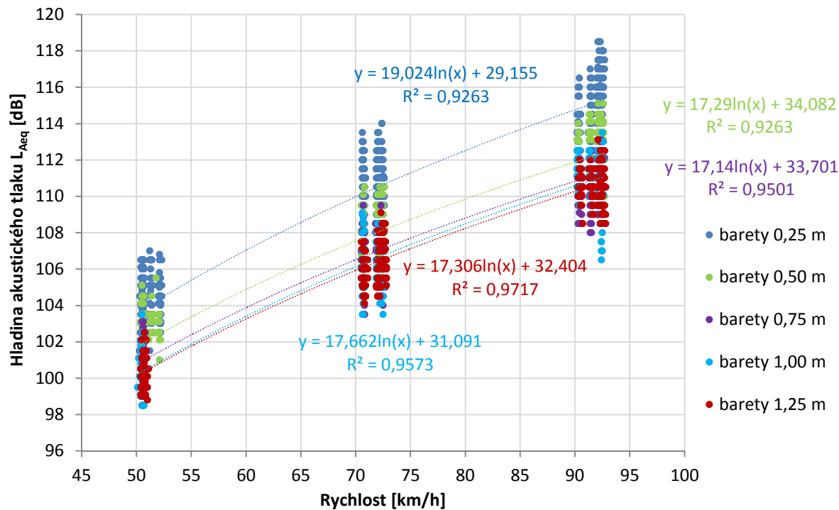
Graf 30: Hodnoty L_{Aeq} vzorků VDZ
