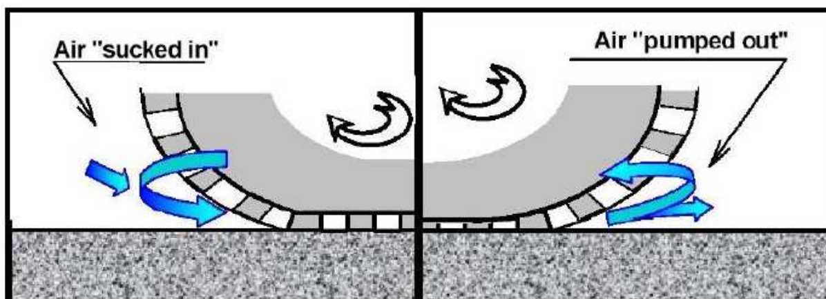
Obrázek 5: Znárodnění sání a pumpování vzduchu [5]
