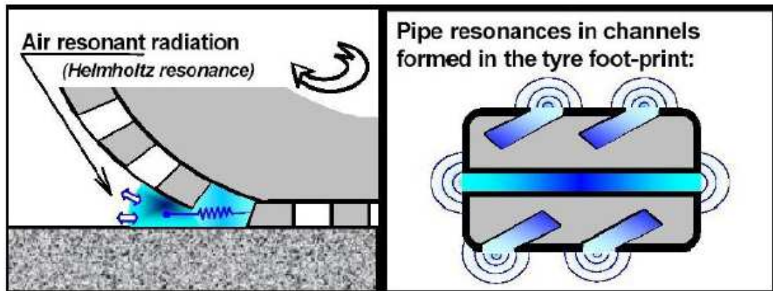
Obrázek 9: Schéma rezonátoru [5]
