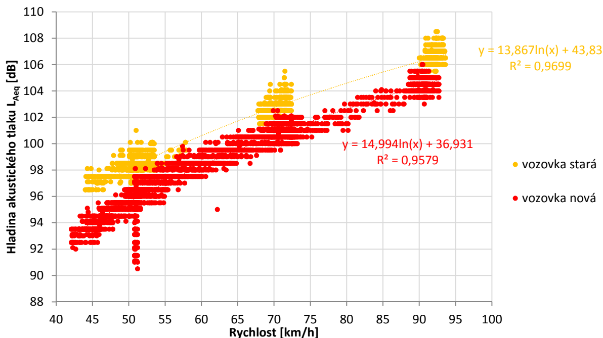
Graf 31: Hodnoty L_{Aeq} vzorků vozovek
