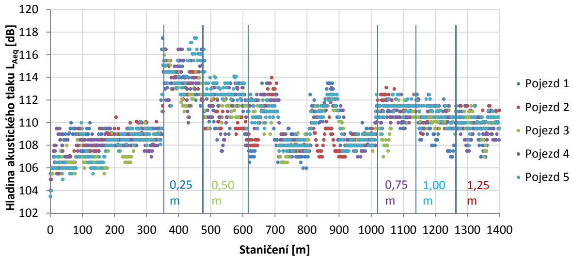
Graf 18: Průběh L_{Aeq} v závislosti na staničení (90 km/h)
