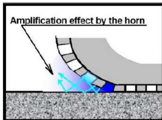
Obrázek 8: Trubkový efekt vytvořený pneumatikou [5]
