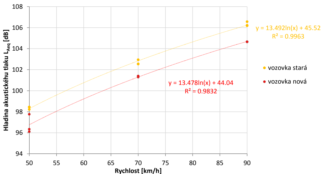
Graf 13: Průměrné hodnoty hladiny akustického tlaku vozovek
