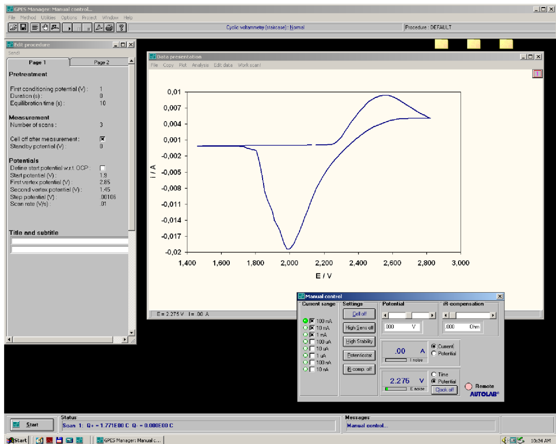
Obr. 22: Výsledek měření na profesionálním přístroji AUTOLAB PGSTAT 12
