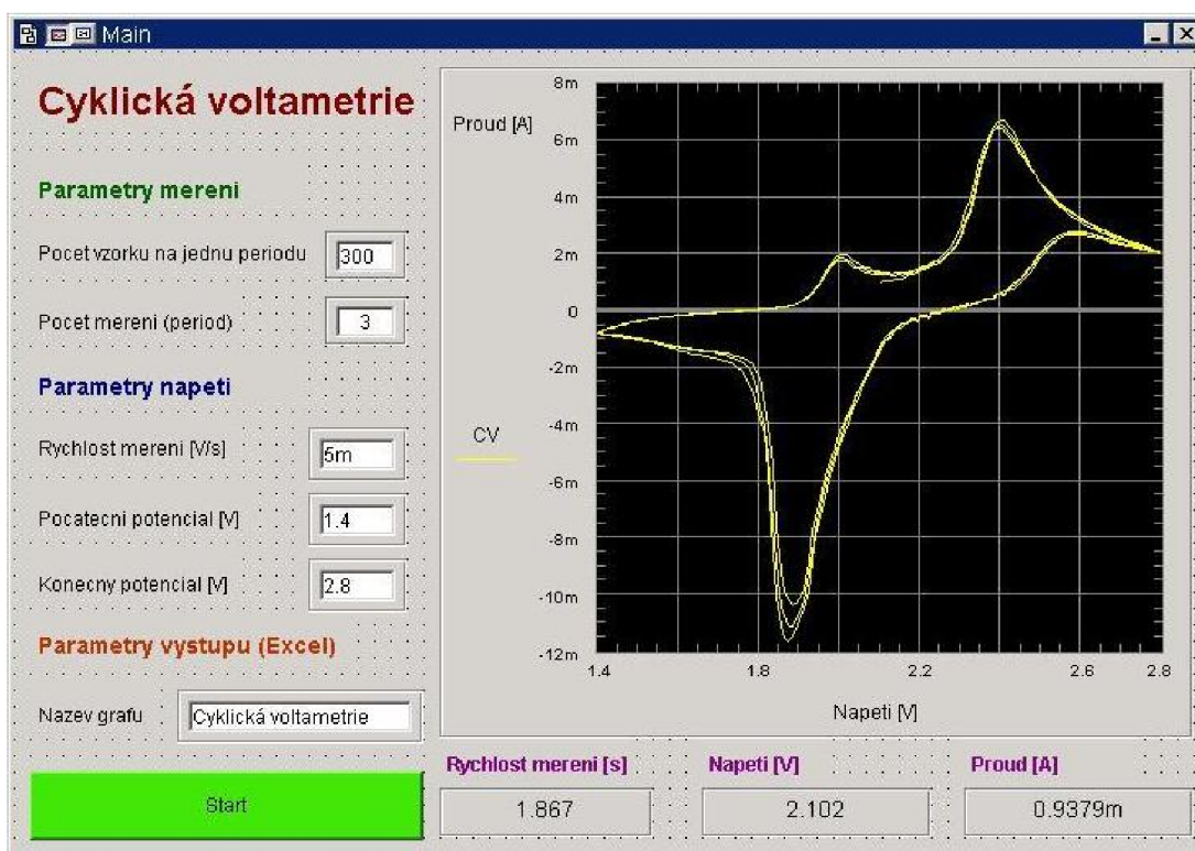
Obr. 20: Ovládací panel měřicí aplikace
