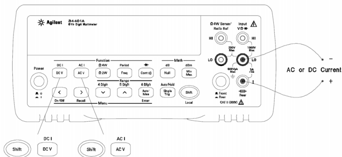
Obř. 10: Přední panel multimetru Agilent 34401A, zapojení pro měření proudu
