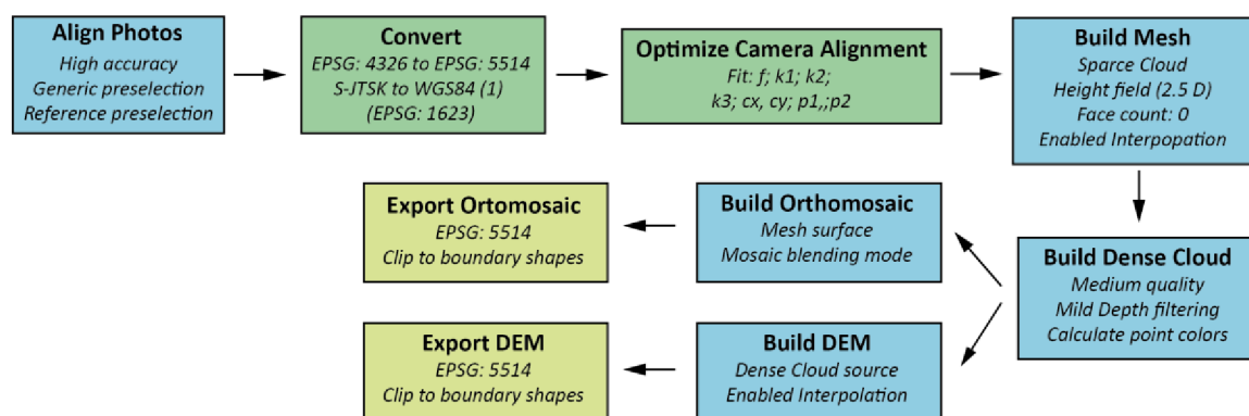
Obr. 14 Schéma postupu pro vytvoření ortomozaiek a DEM
