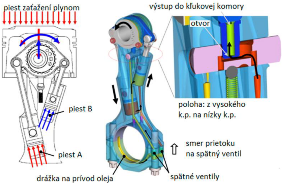
Obr. 15 - Znázornenie hydraulického okruhu a 3/2 ventilu ojnice [11]
