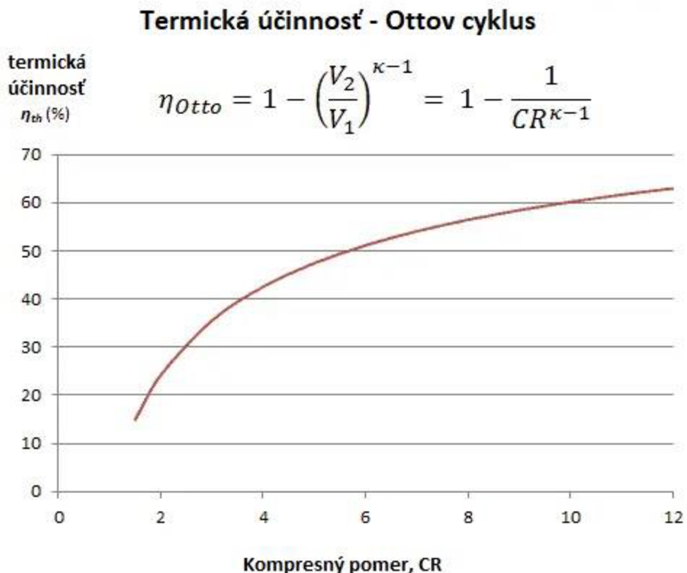
Obr. 1–Závislosť termickej účinnosti na kompresnom pomere u zážihového motora [2]
