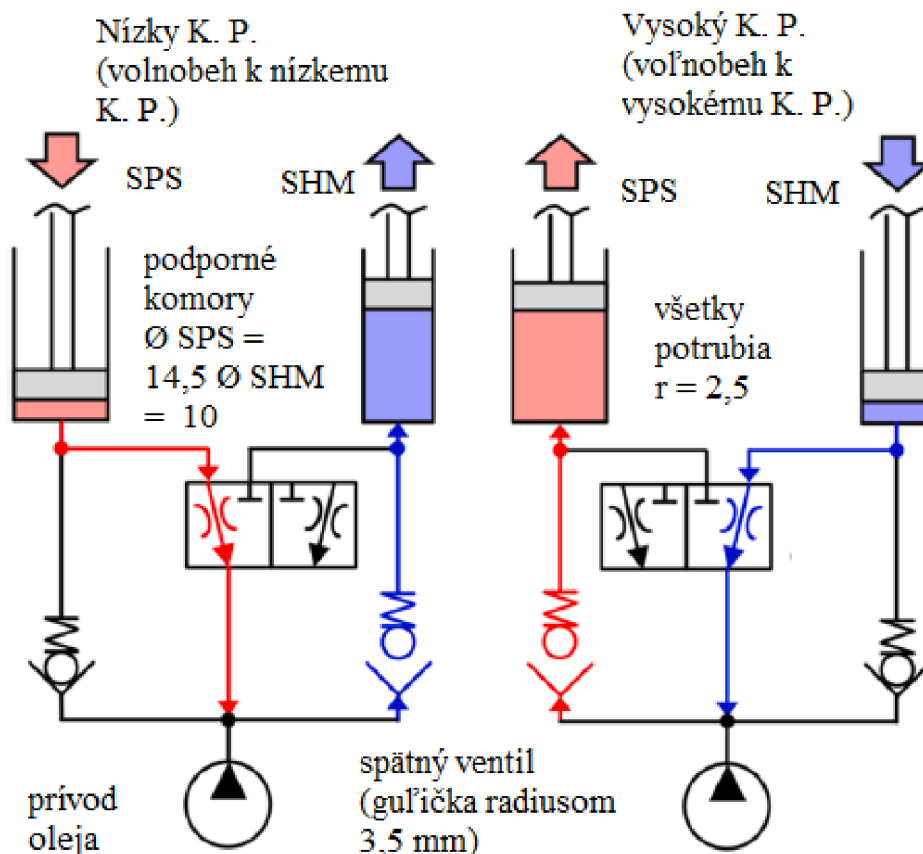
Obr. 16 - Hydraulické parametre ojnice VCR skúmané v tejto práci, rozmery v mm
