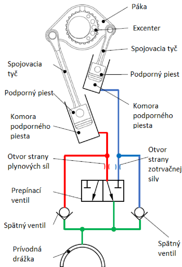
Obr. 12 - Podporný mechanizmus a hydraulický obvod ojnice VCR
