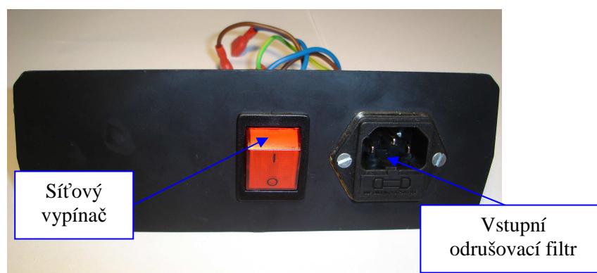
Obr. 20 Uspořádání jednotlivých částí zdroje na zadním panelu
