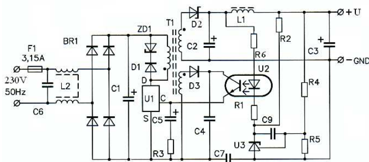
Obr. 15 Zpětná vazba s optronem a obvodem TL431 (převzato z [1])
