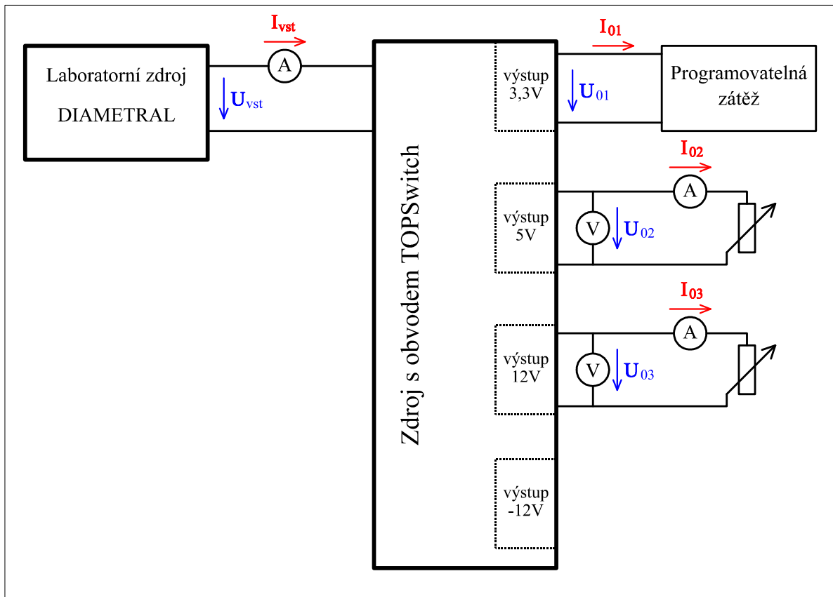
Obr. 22 Měřicí zapojení zdroje
