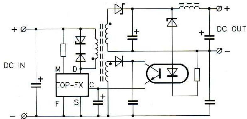
Obr. 7 Typické aplikační zapojení blokujícího měniče s obvodem TOPSwitch-FX (převzato z [1])
