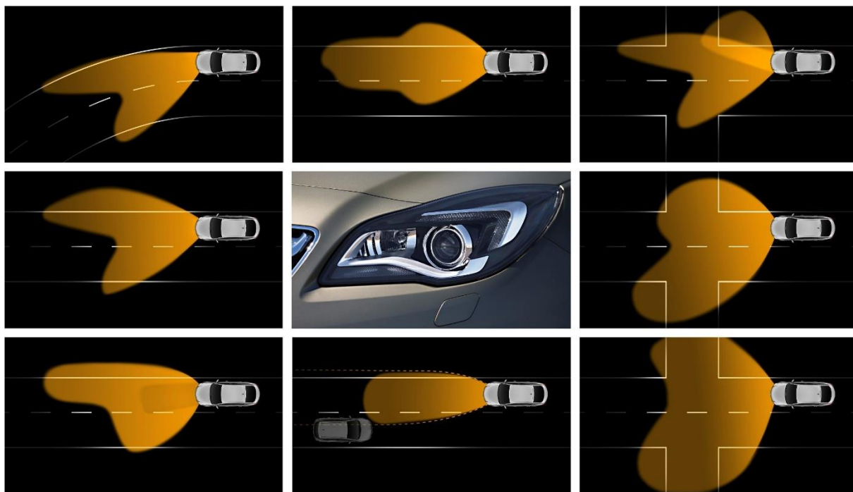
Obr. č. 10 - Adaptivní světlometry [26]
