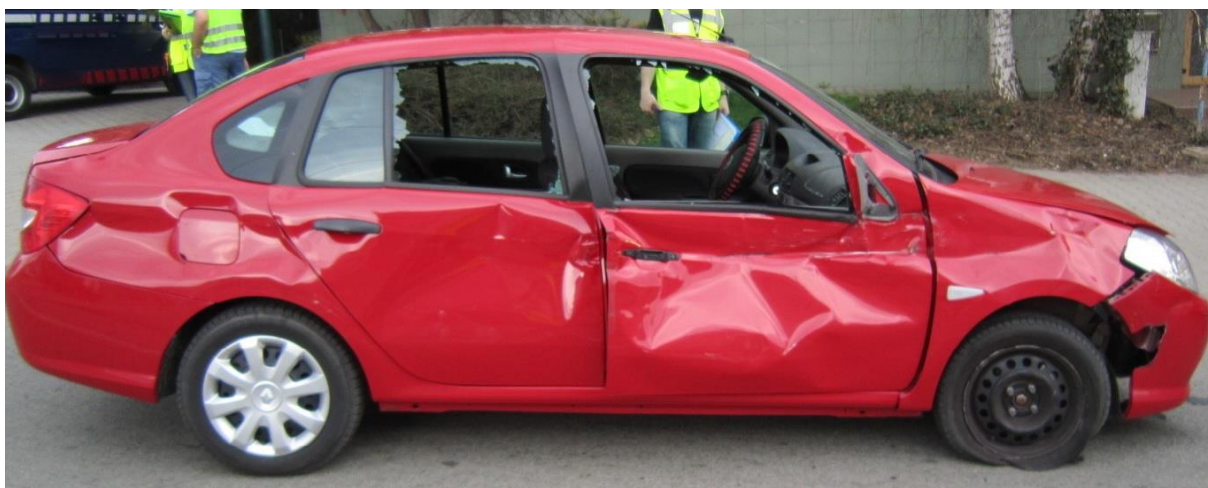
Obr. č. 14 - Poškození vozidla po střetu s kolejovým vozidlem
