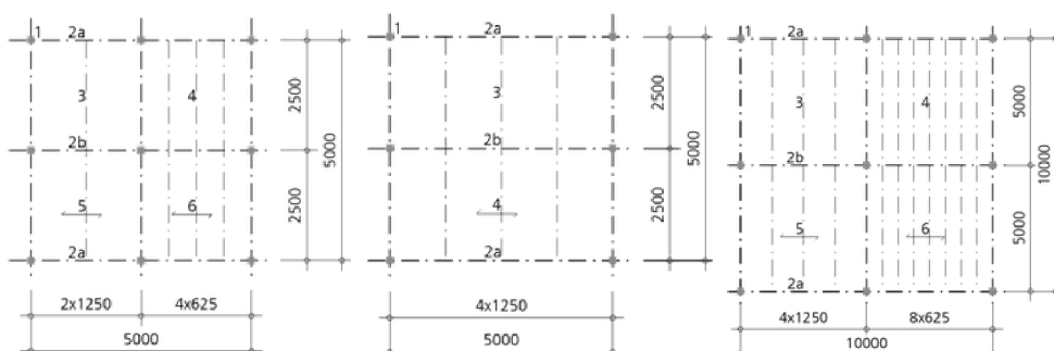
Obr. 14 Půdorysné rastry těžkého skeletu (Kolb, 2011)
