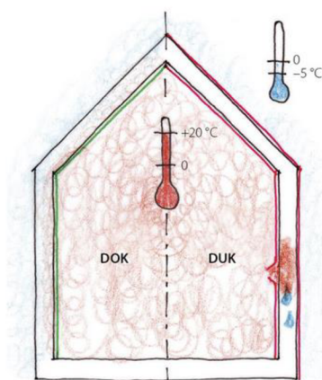
Obr. 23 Difuzně otevřená/uzavřená stavba (Růžička, 2014)
