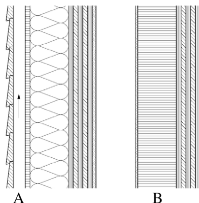
Obr. 6 A – Skladba stěny CLT s provětrávanou fasádou B – Skladba stěny CLT s kompaktní fasádou (Kolb, 2011)
