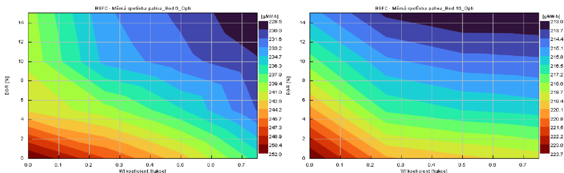
Obr. 16: EGR vs. vodní vstřikování – měrná spotřeba paliva
