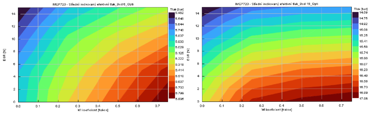
Obr. 12: EGR vs. vodní vstřikování – střední efektivní tlak
