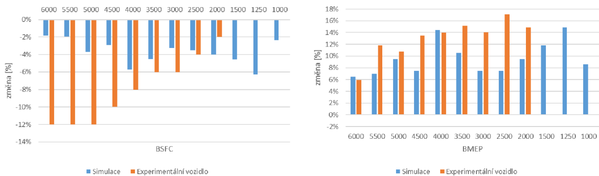
Obr. 22: Relativní srovnání simulace a experimentu (BSFC, BMEP)
