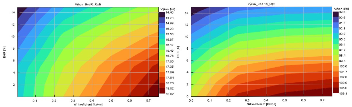
Obr. 13: EGR vs. vodní vstřikování – výkon
