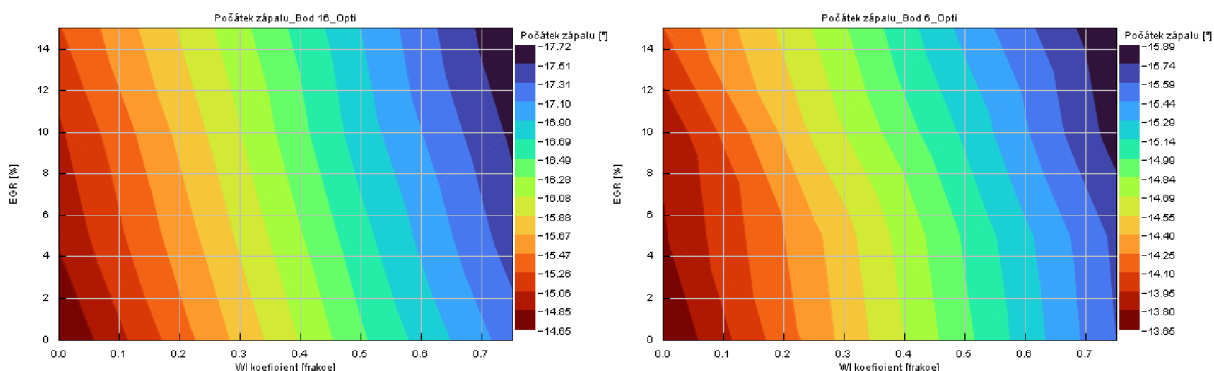
Obr. 10: EGR vs. vodní vstříkovaní – počátek zápalu
