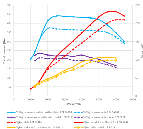
Obr. 20: Změřená data experimentálního vozidla s motorem 2.0 l EA888 a modelem 1.5 l EA211 evo
