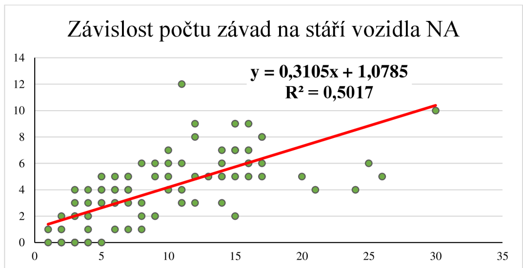
Obrázek 49 - Graf závislosti počtu závad na stáří vozidla
