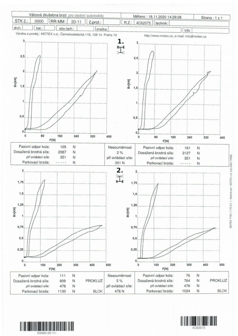
Obrázek 20 - Záznam z válčové zkušebny brzd [9]
