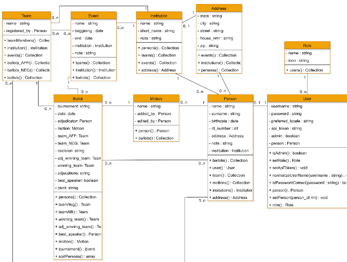
Obrázek 14 - Diagram tříd
