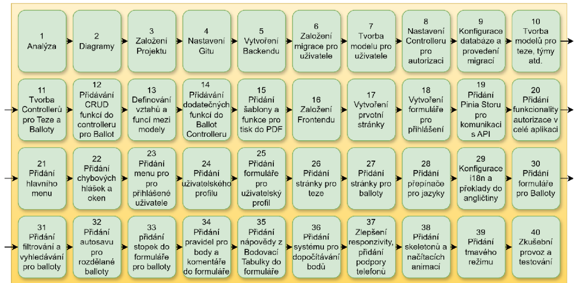
Obrázek 13 - Workflow Diagram
