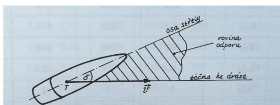
Obrázek 4. Úhel náběhu měřený v rovině odporu 18
