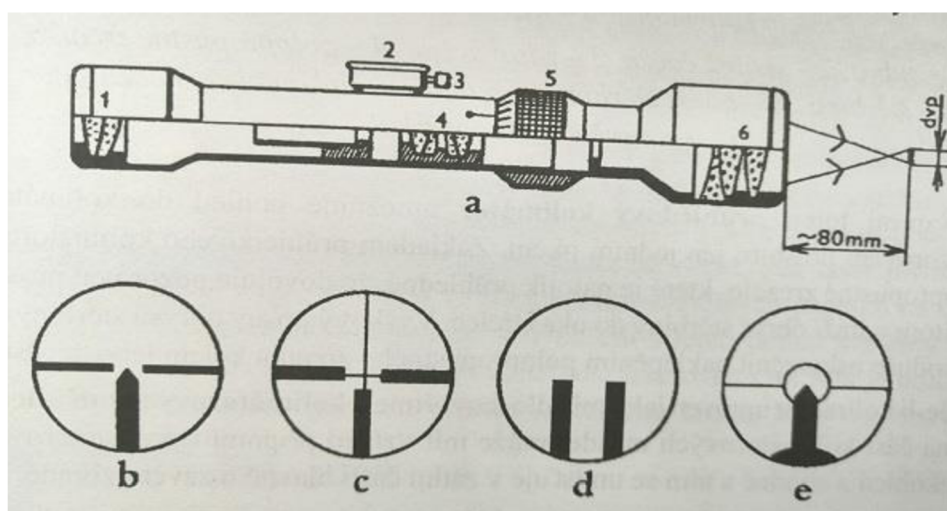
Obrázek 9. Zaměřovací dalekohled 25
