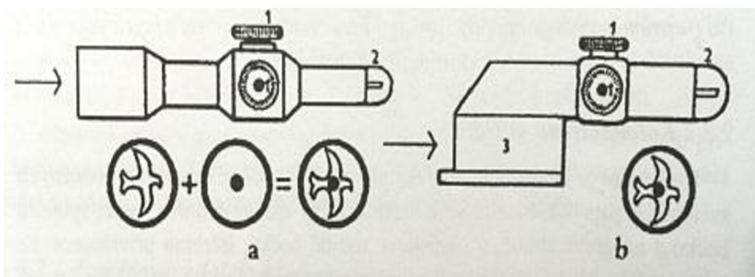
Obrázek 10. Kolimátorová mířidla 26
