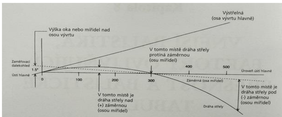
Obrázek 1. Dráha střely 8
